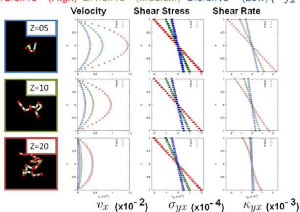
図 5.5 線形のからみあい高分子( Z=5, 10, 20 )の場合の三つの異なる圧力勾配下における速度場 V_x 、せん断応力 \sigma_{yx} 、せん断速度 \kappa_{yx}
