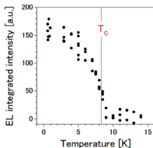
図 4-5-1-2. 図 4-5-1-1 で測定したエレクトロルミネッセンス積分強度を温度に対してプロットした図。Nb 電極が超伝導体に転移する臨界温度 8.3K より低い温度で、発光強度の急激な増加が観測された。
