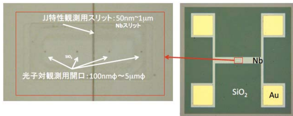
図 4-6-3-1Nb/n-InGaAs/p-InGaAs/Nb 構造 LED の表面 Nb 電極と、光子対観測用開口部分の拡大 SEM 写真。
