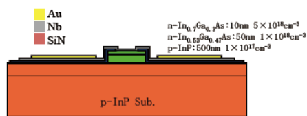
図 4-4-1-3 シングルヘテロ接合デバイス
