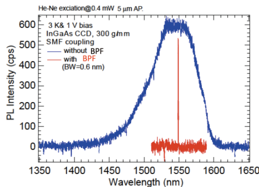
図 4-6-3-3 Nb/n-InGaAs/p-InGaAs/Nb 構造 LED の発光スペクトルと、バンド幅 0.6\text{nm} のバンドパスフィルターを用いて測定したシャープな発光線。
