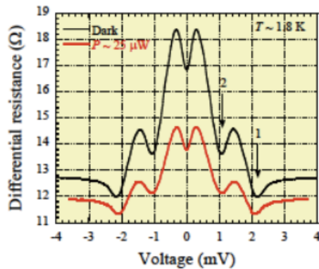
図 4-3-1-4 光照射前後の微分抵抗特性 (赤線が 25 \mu W 光照射時)
