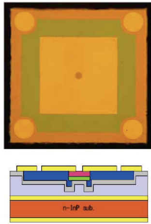
図 4-6-2-4 Au 電極基板貼り付けデバイスの表面写真と断面構造。
