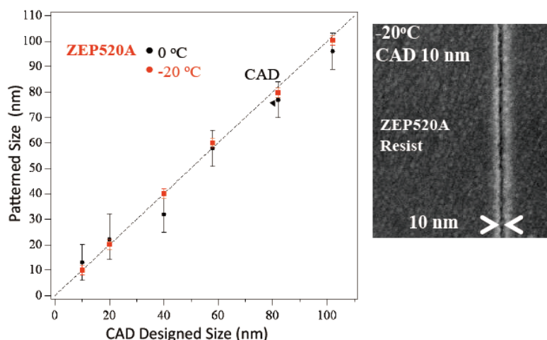
図 4-2-4-1 電子ビームレジスト ZEP520A の現像温度を下げる（CTD: Cold-Temperature Development）方法により、レジストパターニングの解像度が大幅に向上する。
