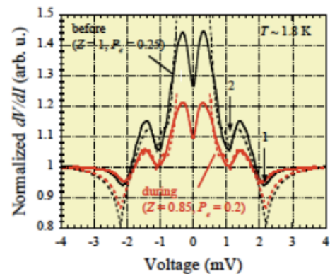
図 4-3-1-5 光照射前後の微分抵抗特性と 超伝導近接効果理論との比較（黒破線、 赤破線がそれぞれ光照射無し、有り時の 特性のモデルフィッティング）。
