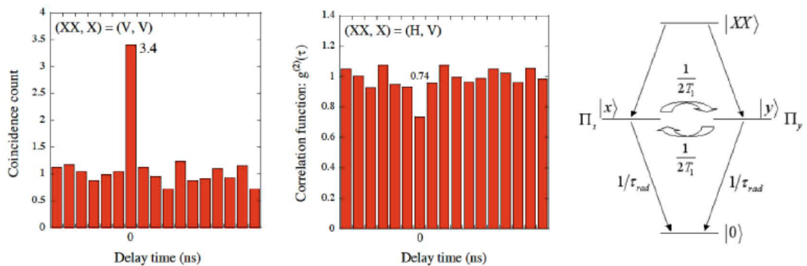
図 4-1-3. 偏光状態を考慮した励起子分子(XX)と励起子(X)発光の光子相関測定結果と、異なるスピンを持つ励起子状態間のスピン反転の模式図。励起子分子(XX)から直線偏光した光子放出によって2つの励起子スピン状態が生成するが、寿命 \tau_{\text{rad}} で発光する前に、その状態間でスピン緩和時間 T_1 でスピン反転する可能性を示す。
