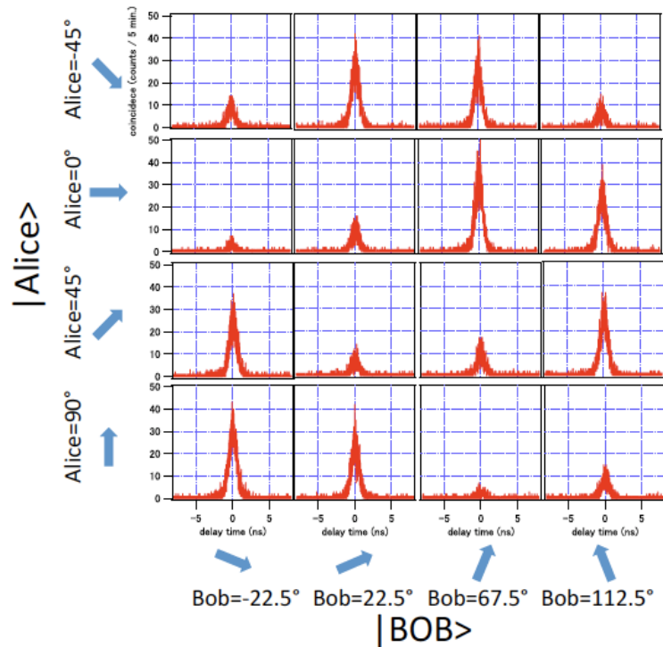
図 4-6-3-5 Alice の 4 種類の偏光、Bob の 4 種類の偏光の組み合わせ 16 通りについての光子偏光相関測定結果。
