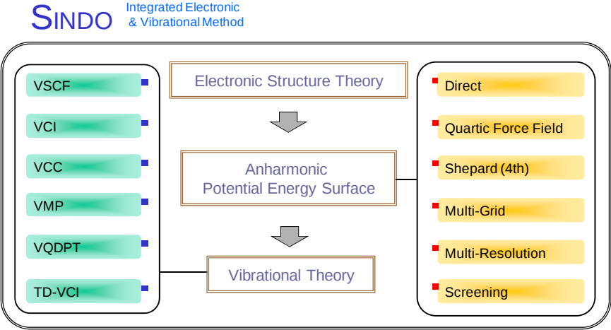
図 3.6. SINDO プログラムの構成.
