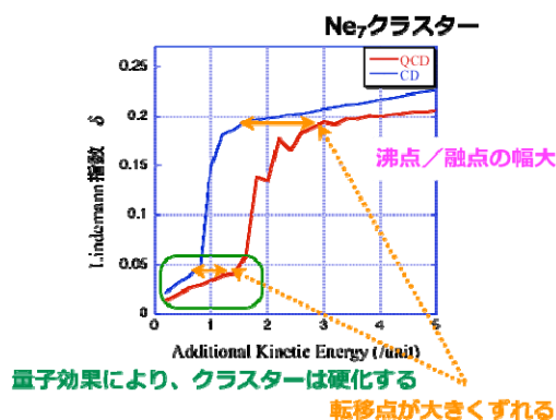
図 3.8. \text{Ne}_7 クラスターの構造相転移の様子.
