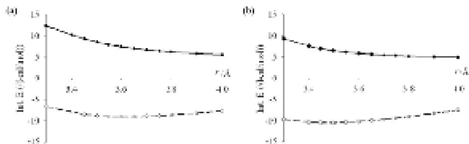
図4.10. (a) [H-Cu^{2+}-H] および(b) H-H_2-H の面間距離とスタッキングエネルギーの関係. 実線が通常の DFT で計算した結果 で, 破線が ALL 汎関数の補正を入れた結果である.
