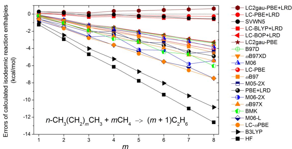
図 4.2. 各 DFT 計算によるアルカンの isodesmic 反応の反応エネルギー計算値の誤差。
