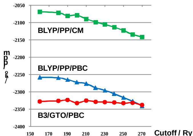
図 1.5. \text{VOCl}_3 結晶の ^{51}\text{V} の核磁気遮蔽定数計算値の平面波のカットオフ値に対する収束性.
