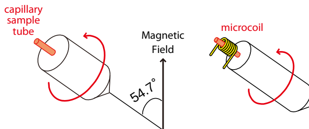
図 10: Piggy-back 方式によるマイクロコイル MAS の模式図。既存の MAS 用試料管にキャピラリー試料管を突き立てて回転させ(左)、回転するキャピラリー部分のみマイクロコイル内に収める(右)。
