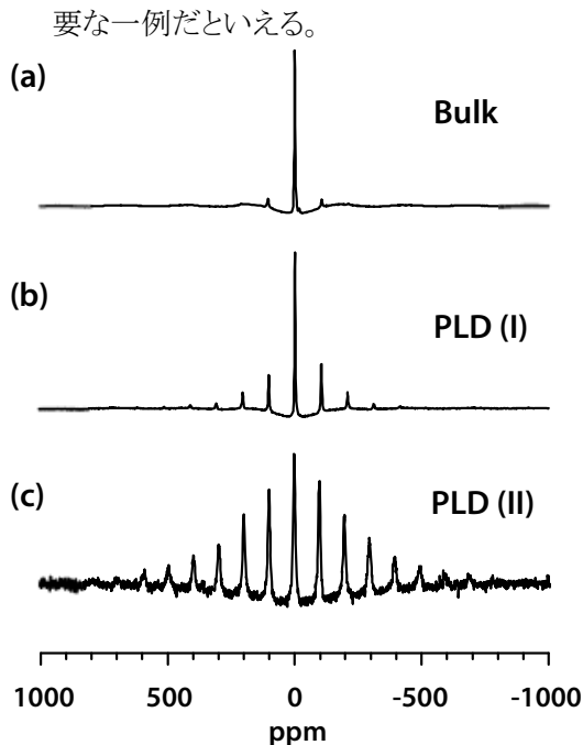
図 13: 7T の磁場下で測定した \text{LiCoO}_2 の ^7\text{Li} マイクロコイル MAS スペクトル。(a)は原材料のスペクトル。(b)および(c)は PLD 法によりガラス基板上に作製した薄膜試料から削り取った粉末試料のスペクトル。(b)と(c)では PLD 時のガラス基板の温度、および PLD 後の熱処理の仕方に違いがある。いずれの薄膜試料も、バルク状態とは異なるスペクトルを示しており、特異な構造を形成していることが示唆される。
