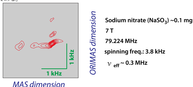
図 25: 亜硝酸ナトリウム粉末における、 23 Na 核の ORIMAS スペクトル。マイクロコイル MAS を利用して測定。
