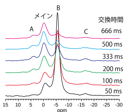
図 9: B の位置の cross section スペクトルの交換時間依存性
