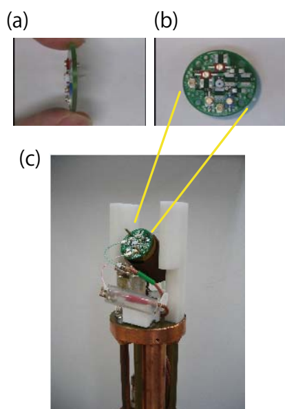
図 11: コイン型マイクロコイル MAS プロブの (a) 側面図および (b) 正面図。 (c) 前川グループ所有の 4mm MAS プロブにコイン型マイクロコイル MAS プロブを装着したところ。
