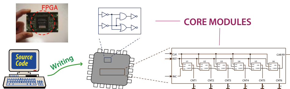
図 18：FPGA の一例（写真）と、プログラミングの概念図（イラスト）。デジタル回路をハードウェア記述言語により構築し、書き込むことにより、カスタマイズされた LSI が完成する。
