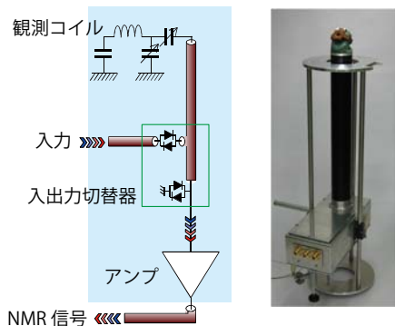
図1: (左) 検出器冷却プローブの模式図、(右) 作製したプローブの外観
