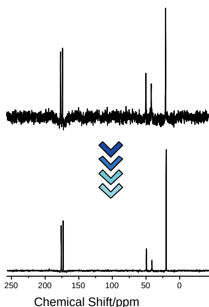
図 5: 位相共分散処理によるノイズ除去結果
