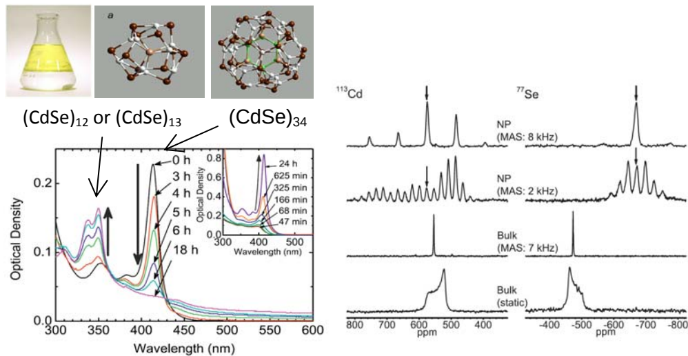
図 31: 溶液中で大量合成された CdSe ナノ粒子とその ^{113}\text{Cd} , ^{77}\text{Se} NMR スペクトル
