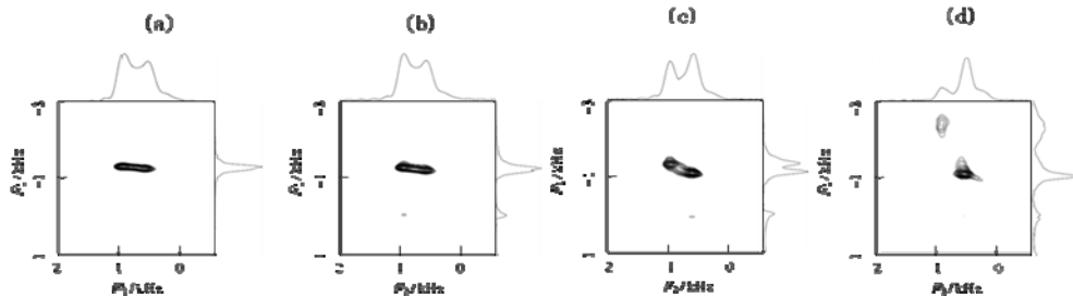
Fig. 37: 振幅不完全性のシミュレーション結果. (a) 理想パルス. (b) 不完全性 25%, (c) 不完全性 50%, (d) 不完全性 75%.
