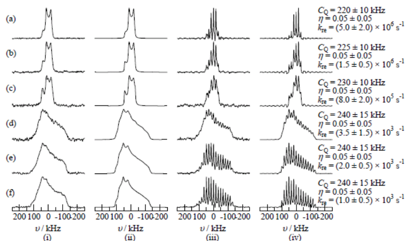
Fig. 42: \text{CoSiF}_6 \cdot 6\text{H}_2\text{O} の ^2\text{H} NMR スペクトルの温度依存性. (i), (iii)はそれぞれエコー法と本法(Fig. 5(b))で測定したスペクトルを表わす.(i, iii) 実測, (ii, iv) シミュレーション.
