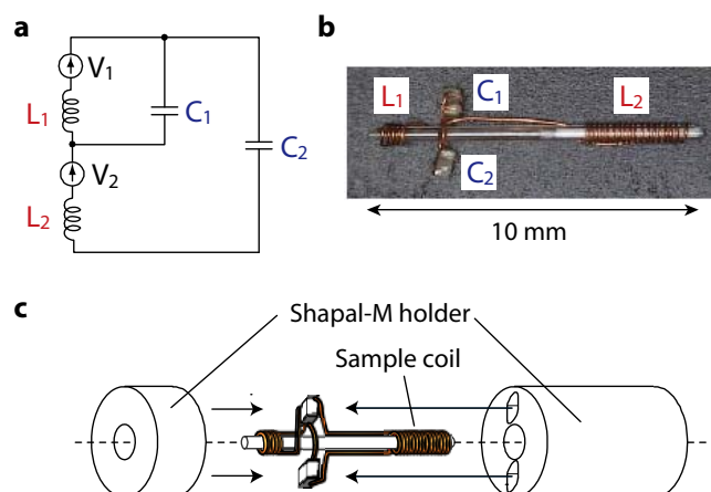
図 15: (a) 二重共鳴 MACS 共振器の回路図と(b)現物の写真。V1 および V2 はそれぞれ一次コイルとの相互誘導結合による起電力を表している。また、コイル L2 が試料用マイクロコイルの役割を果たしており、ここに微量粉末試料が入る。この二重共鳴 MACS 共振器を、(c)に示すようにホルダー(マシナブルセラミックス、Shapal-M で作製)にセットしてローターに挿入し、コイル・試料回転を行う。
