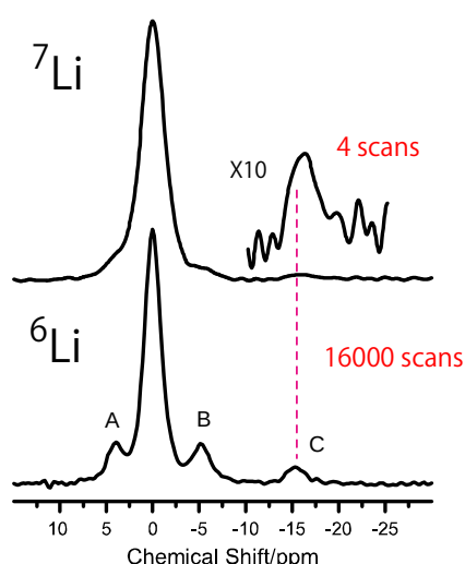
図 7: ^7\text{Li} と ^6\text{Li} の固体高分解能 NMR スペクトルの比較。試料: \text{LiCoO}_2
