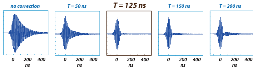
図 22: 能動制御を用いた、ガウス関数を包絡線とするラジオ波パルスの生成実験。回路の共振周波数と Q 値から求まる時定数 T=125\text{ns} を用いて設計したパルスが、意図した通りの包絡線を生成している。
