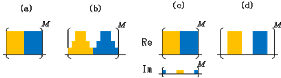
Fig. 36: パルス不完全性の種類. (a) 完全なパルス, (b) 振幅の不完全性, (c) 位相の不完全性, (d) 有限のパルス切り替え時間.
