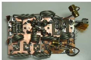
図 29: duplexer 写真
