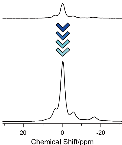
図2: (上) 市販プローブ、(下) 検出器冷却プローブで測定したLiCoO 2 の 6 Li固体高分解能スペクトル。
