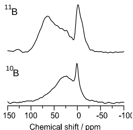
図4: ボロンドープダイヤモンドの ^{11}\text{B} と ^{10}\text{B} のNMRスペクトルの比較
