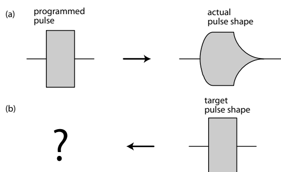
図 21 : (a) 例として、矩形のラジオ波パルスを生成しても (左)、実際にコイル内で発生するラジオ波パルスの包絡線に過渡現象が現れる (右)。(b) そこで発想を逆転させて、実際に核スピンス系に照射するパルス波形から、プログラムすべきパルス波形を逆算するアプローチを取る、過渡現象の能動制御の発想を取り入れた。
