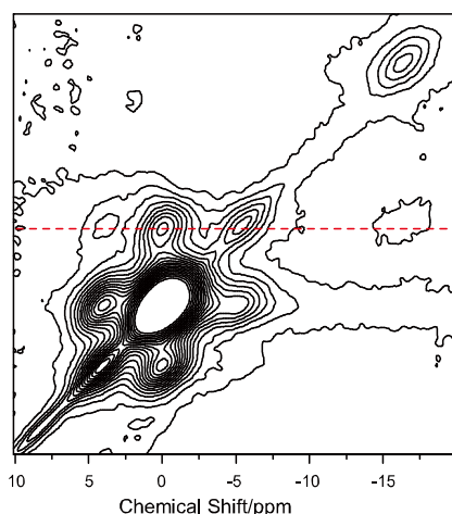
図 8: \text{LiCoO}_2 の二次元 ^6\text{Li} - ^6\text{Li} 相関 NMR スペクトル。交換時間は 333ms であり、点線で示したサイト B の位置の cross section スペクトルの交換時間依存性を図 9 に示した。
