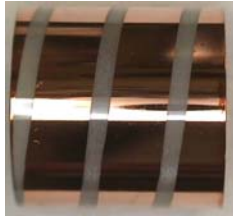
図 27: サファイヤにメッキ形成したコイル
