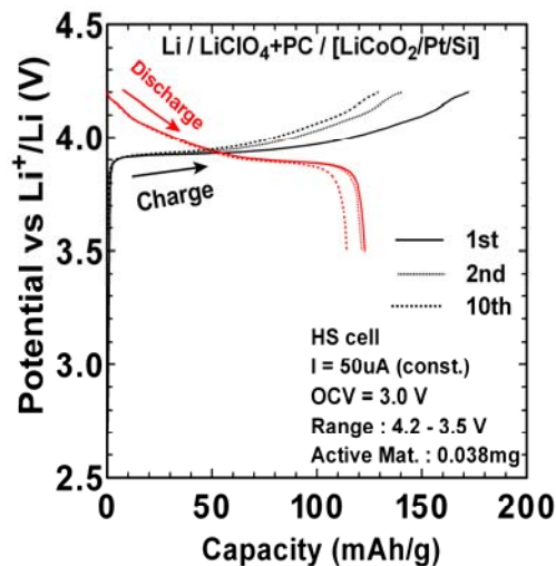
図 35 PLD 薄膜正極を用いたリチウムイオン電池の充放電特性
