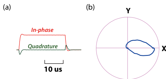
図 17：ピックアップコイルを用いて検出した、Q 値 100、周波数 100 MHz の共振回路内におけるパルスの応答。(a) 直交復調によって、in-phase 成分と quadrature 成分をプロットした図と (b) その極座標表示。
