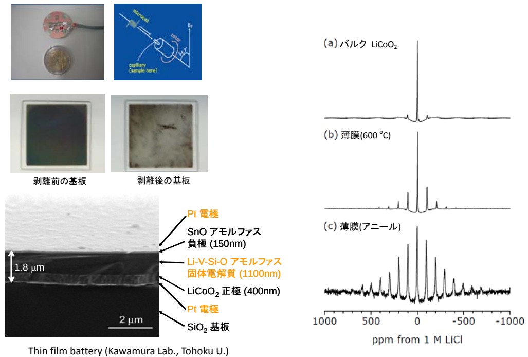
図 34: 7T の磁場下で測定した \text{LiCoO}_2 の ^7\text{Li} マイクロコイル MAS スペクトル。(a)は原材料のスペクトル。(b)および(c)は PLD 法によりガラス基板上に作製した薄膜試料から削り取った粉末試料のスペクトル。(b)と(c)では PLD 時のガラス基板の温度、および PLD 後の熱処理の仕方に違いがある。いずれの薄膜試料も、バルク状態とは異なるスペクトルを示しており、Li イオン脱離に伴う Co イオンの価数変化が起きていると考えられる。
