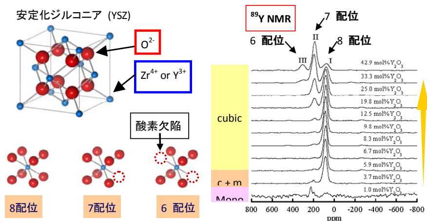
図 30: イットリア安定化ジルコニアの ^{89}\text{Y} MAS-NMR スペクトルによる酸素欠陥同定結果
