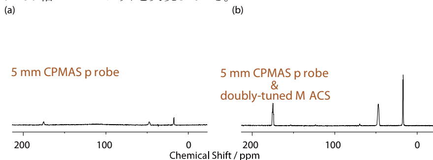
図 16 : 0.1mg ^{13}\text{C} ラベル粉末アラニンの CPMAS スペクトル。測定磁場は 7T で試料回転速度は 10kHz。(a)は市販の 5 mm CPMAS プローブを用いて測定したスペクトル。(b)は同一プローブ、同一試料を用いて二重共鳴 MACS 法を行い得られたスペクトル。
