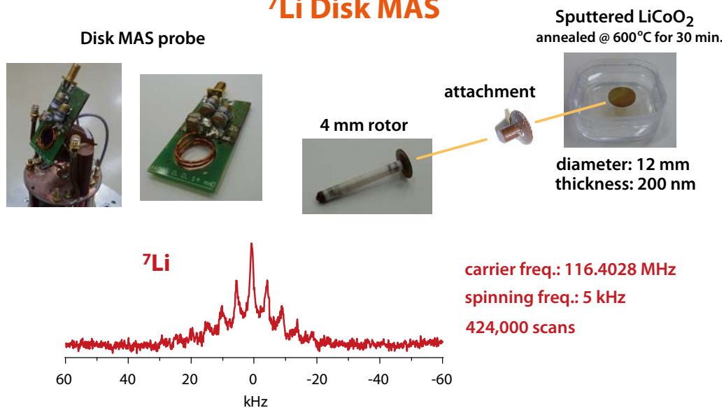
図 26: 薄膜試料の ex-situ キャラクタリゼーションのために開発した、Disk MAS 法の概略。
