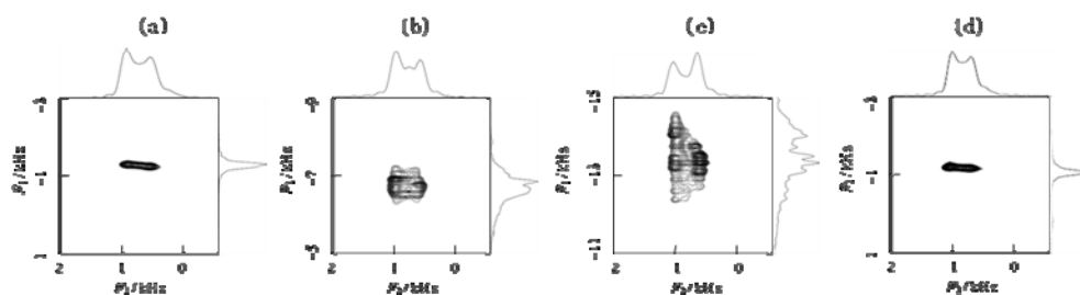
Fig. 38: 位相不完全性のシミュレーション結果. (a) 理想パルス. (b) 1°の位相のずれ (c) 2°の位相のずれ. (d) 逆順の 5°の位相のずれ
