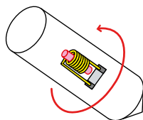
図 14: MACS 法の模式図。この方式では、MAS 用試料管に共振をとったマイクロコイルを挿入し回転させる。ラジオ波パルスの送信・NMR 信号の受信はワイヤレスで通常の MAS プローブを用いて行う。
