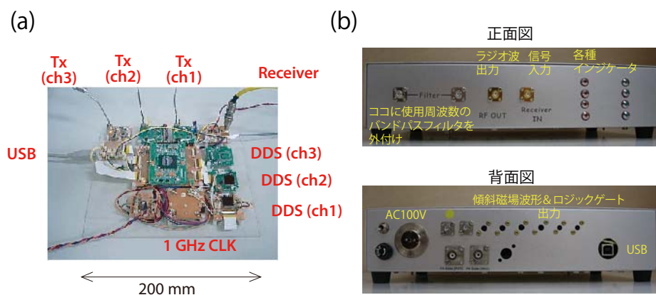
図19：FPGA 集約型分光計（OPENCORE NMR 分光計）の概観。(a) シャーシなしタイプ、および(b) シャーシありタイプ。
