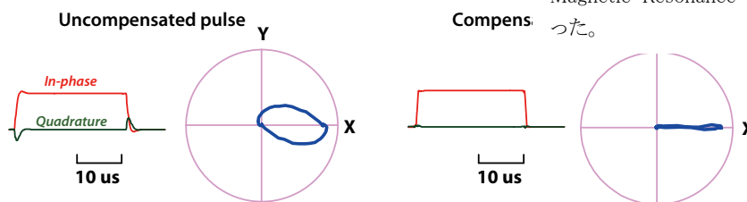
図 24: (左) 能動制御を行わない場合と(右)行った場合のラジオ波パルスの in-phase と quadrature 成分、およびその極座標プロット。
