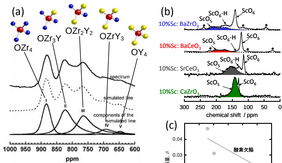
図 33: (a) Y ドープセリア試料の ^{17}\text{O} MAS NMR スペクトル, (b) Sc ドープ \text{BaZrO}_3 、 \text{BaCeO}_3 、 \text{CaZrO}_3 、および \text{SrCeO}_3 の Sc-45 MAS-NMR スペクトル, (c) Sc 周囲の酸素空孔濃度とプロトン性欠陥濃度の四重極結合定数依存性
