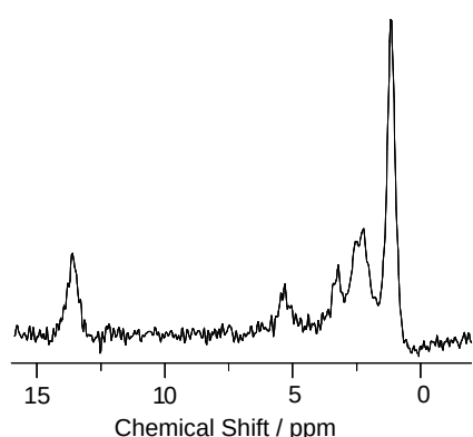
図 3: 天然存在比の天然存在比の ^2\text{H} の固体高分解能スペクトル (試料: dimedone)
