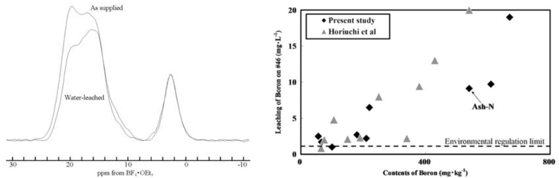
図 32: 火力発電所から排出された石炭灰(Ash-N)の ^{11}\text{B} NMR スペクトルと灰中のホウ素濃度
