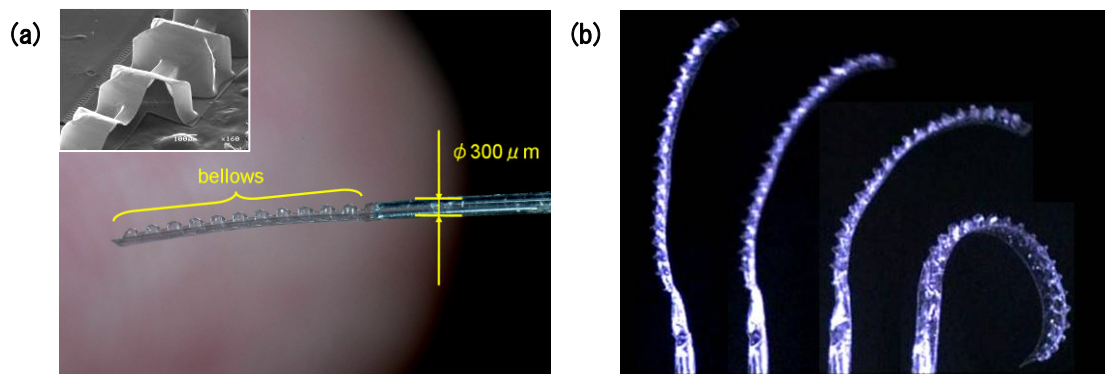
Fig. 4.7.3 (a) 薄膜構造を利用した異方性ベローズを先端部に取り付けた水圧駆動力カテーテル (b) 直径 300\mu\text{m} 、屈曲範囲 0\sim 180^\circ の駆動を実証
