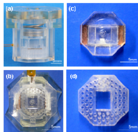
Fig. 4. 3. 2 開発したリアルタイム PCR チップ群 (a) 全体像横から (b) 全体像下面から (c) リアクタ部 (d) スぺーサ部
