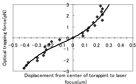
Fig. 4. 1. 3 変位と光トラップ力の関係曲線
