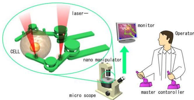
Fig. 4. 1. 1 光駆動ナノマシンによる細胞触診システムのコンセプト
