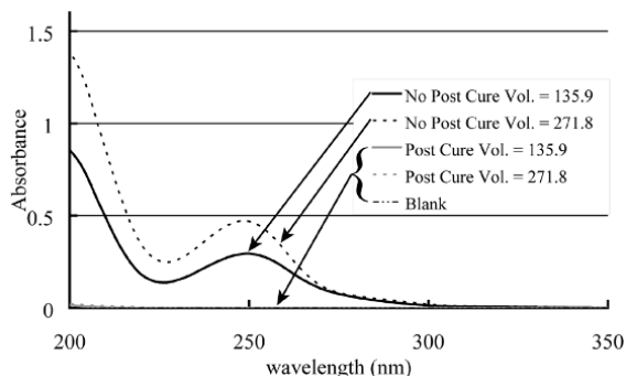
Fig. 4. 4. 4 各ポストベイク条件での溶出物の吸収スペクトル
