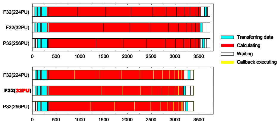
図 3.1-②-4 Ninf-G のタイミングプロファイルとクライアントコールバック機構による高速化(下)
