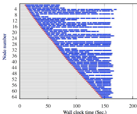
図 3.2-②-2 耐故障性のテスト
