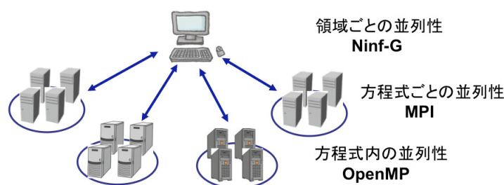
図 3.2-②-1 Ninf-G/MPI/OpenMP ハイブリッドによる並列化
