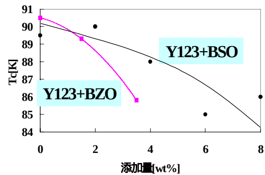
図 53 \text{BaZrO}_3 および \text{BaSnO}_3 添加 Y123 薄膜における添加量と T_c の関係
