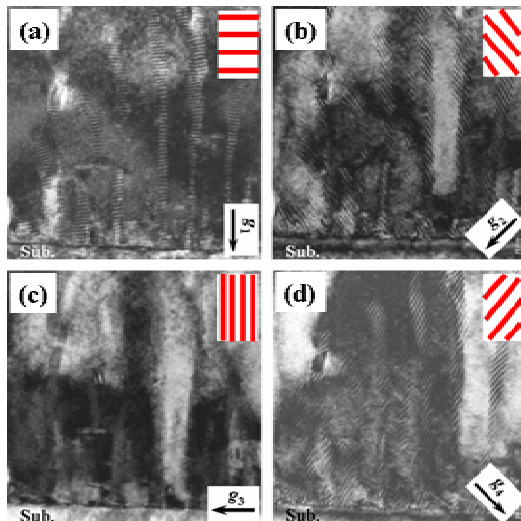
図 35 ナノロッドの縞模様と回折ベクトル ( g_1 \sim g_4 ) との関係を示す明視野像。
