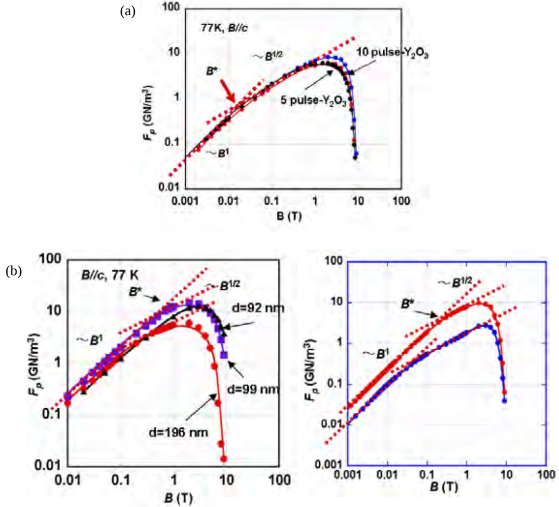
図 6 (a) 転位によるピン止め力, (b) 粒界によるピン止め力, (c) 平行粒界によるピン止め力で、この場合、赤は粒界に平行電流、青は粒界に垂直電流を流したときに対応する。
