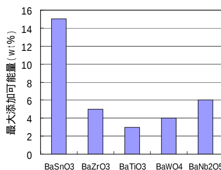
図 50 各種 APC 材料と 90K 以上の T c を示す最大添加量
