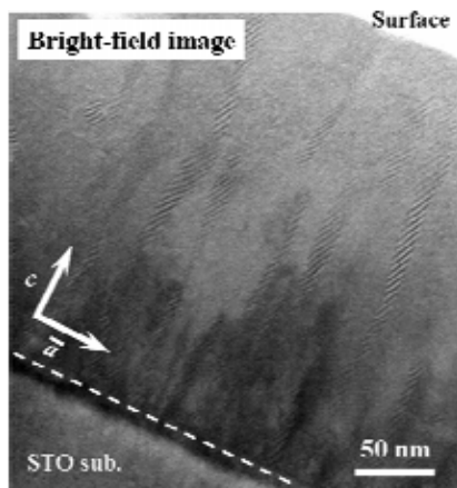
図 32 BaNb 2 O 6 ドーピングEr123 膜に形成されたナノロッドを示す明視野像。
