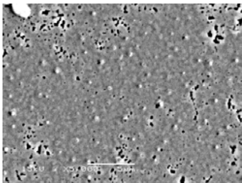
図 40 MOD-Gd123 薄膜表面 SEM 像。
