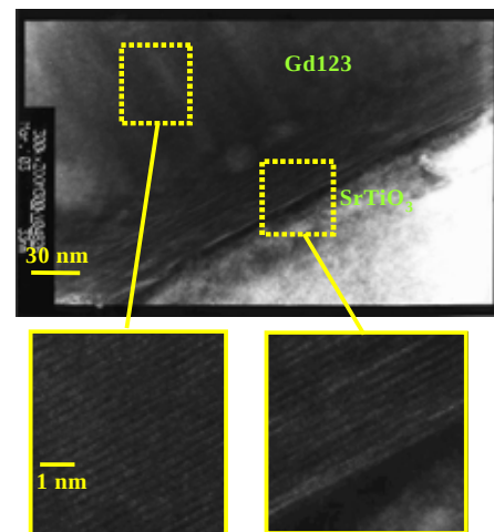
図 46 BaF 2 -Gd123 薄膜断面 TEM 像。
