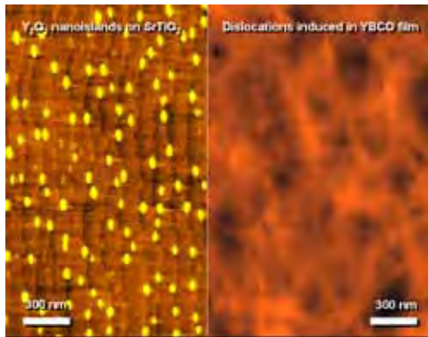
図 9 \text{SrTiO}_3 基板上に形成された \text{Y}_2\text{O}_3 ナノアイランド(左図)。アイランドのサイズは 20～30 nm で \text{SrTiO}_3 基板の原子ステップが見える。右図は導入された YBCO 薄膜中の転位(エッチピット)を示している。
