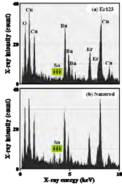
図 28 Er123 相(a)およびナノロッドを含む(b)領域から取得された EDX スペクトル。
