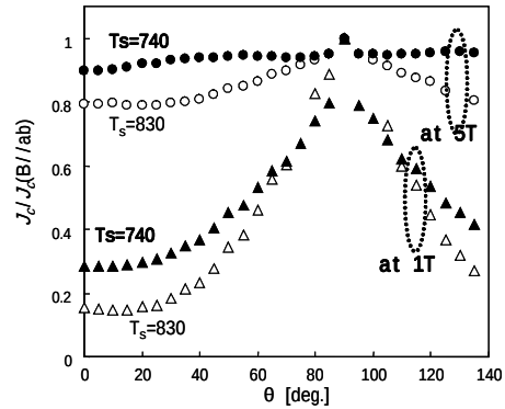
図 18 SmBCO の 77K での J_c 角度依存性
