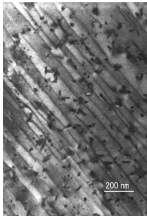
図 57 ナノロッドを含む超伝導膜の平面透過電子顕微鏡像
