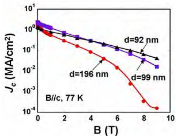
図 13 粒径を変化させた時の GdBCO 薄膜の J_c -B 特性。
