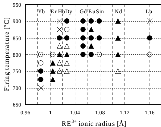
図 39 \text{SrTiO}_3 基板上に作製した RE123 薄膜の結晶配向挙動 (○; c 軸配向膜、●; 面内配向が確認された c 軸配向膜、▲; a 軸配向が混在した c 軸配向膜、△; a 軸配向が混在し面内配向が確認された c 軸配向膜、×; RE123 が成長していないあるいは不純物相が含まれた膜を表す)。
