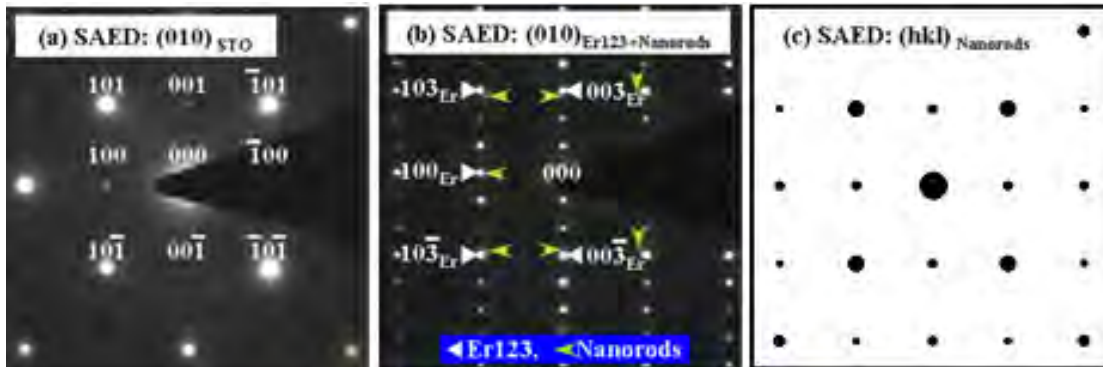
図 29 \text{SrTiO}_3 基板(a)、Er123 相とナノロッドの 2 相領域(b)の制限視野電子回折図形、および(b)からナノロッドの回折斑点を抽出した電子回折図形の模式図。
