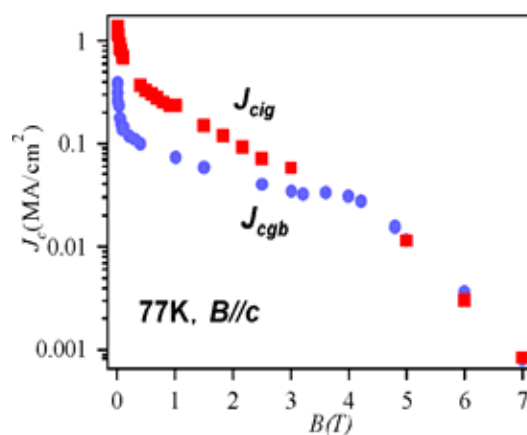
図 86 5 度粒界 J_c(J_{cgb}) と粒界の無い試料の J_c(J_{cig}) の比較。
