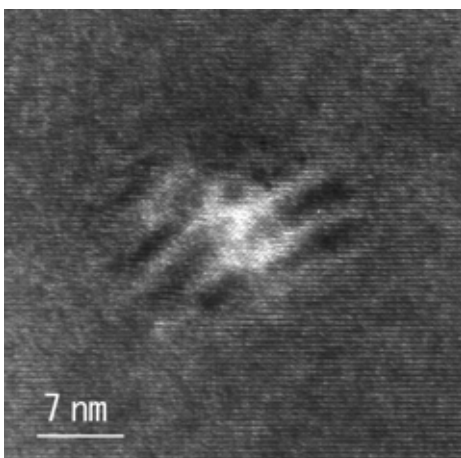
図 58 ナノロッド部分の拡大平面透過電子顕微鏡像
