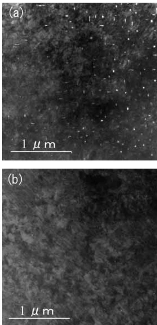
図 65 \text{GdBa}_2\text{Cu}_3\text{O}_y 超伝導膜の平面透過電子顕微鏡像
