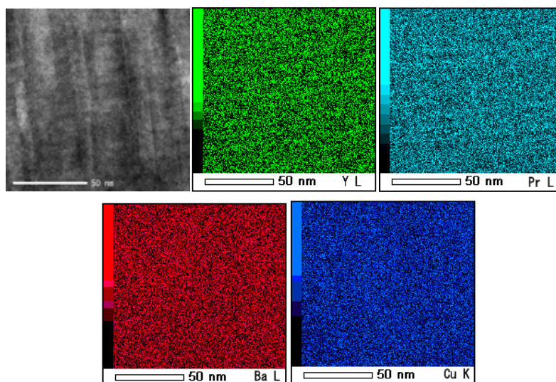
図 66 新規手法による高温超伝導薄膜中の 2 次元 APC 構造。YBa 2 Cu 3 O y (超伝導材料)と PrBa 2 Cu 3 O y (非超伝導材料)の積層構造からなる
