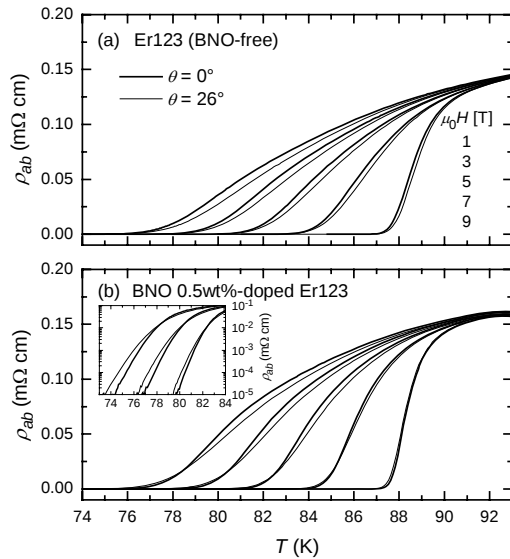
図 84 Er123 および BNO ドープ Er123 薄膜の電気抵抗率の温度依存性。
