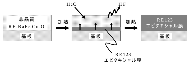
(b) 新しいBaF 2 プロセス(水蒸気導入無し)
