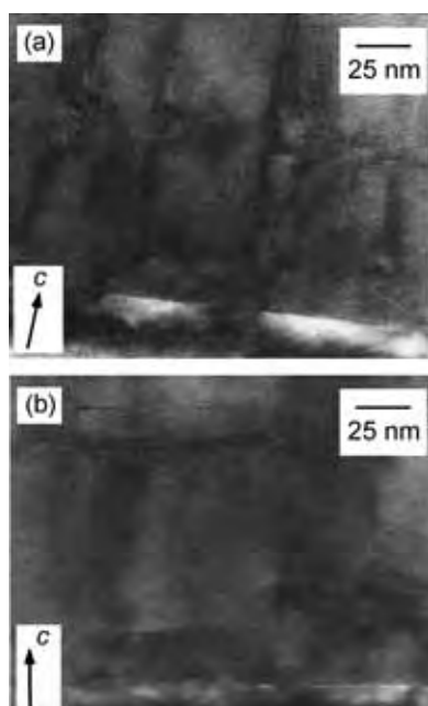
図 79 770 (a)および 850 (b)で成膜した Co0.5%ドープ Er123 薄膜の断面 TEM 像。
