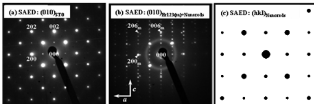
図 34 SrTiO 3 基板(a), Er123 相とナノロッドの 2 相領域(b)の制限視野電子回折図形, および (b)からナノロッドの回折斑点を抽出した電子回折図形の模式図。
