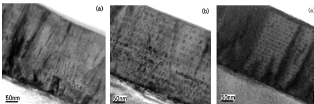
図 62 ナノロッド長を制御した超伝導膜の断面透過電子顕微鏡像
