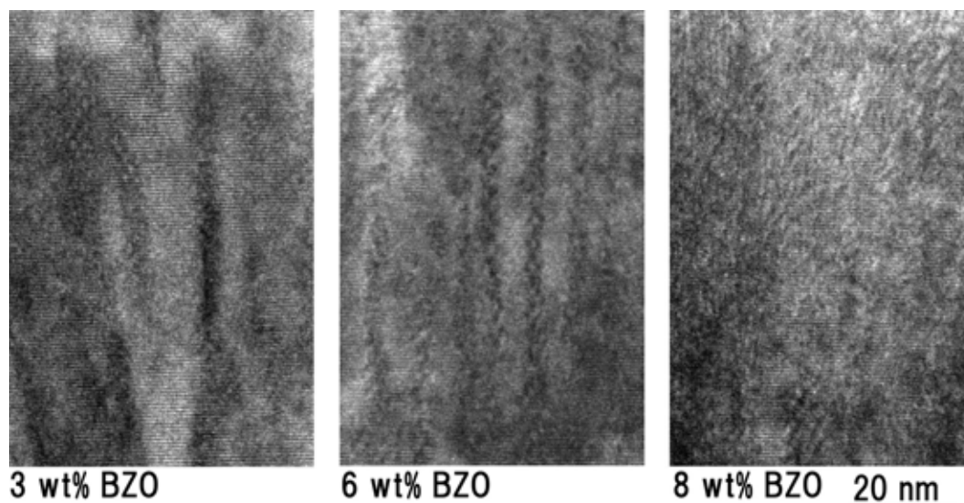
図 63 ナノロッド密度を制御した超伝導膜の断面透過電子顕微鏡像
