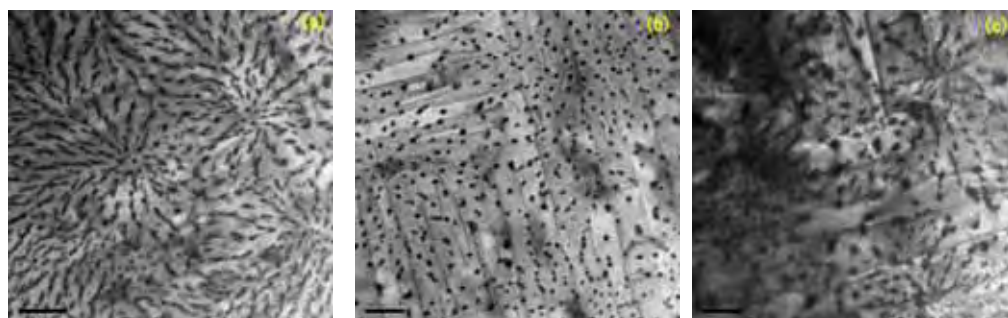
図 61 ナノロッドを含んだ YBCO 膜の平面透過電子顕微鏡像
