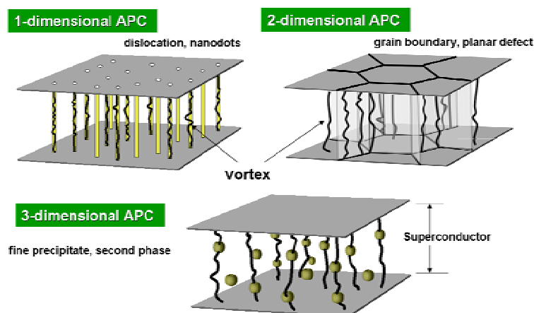
図 2 次元性を考慮した各種の人工ピン構造(1 次元, 2 次元, および 3 次元人工ピン)
