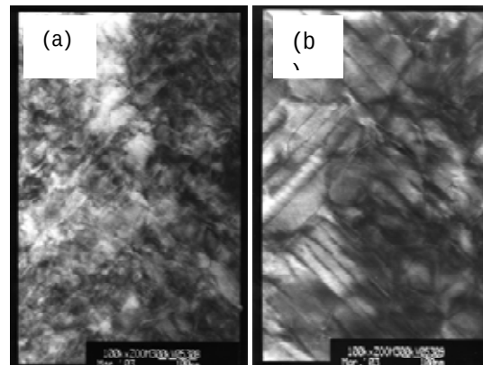
図 78 770^\circ\text{C} (a)および 850^\circ\text{C} (b)で成膜した \text{Co}_{0.5}\% ドープ Er123 薄膜の平面 TEM 像。
