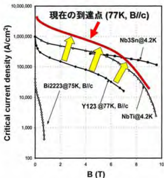
図1 高温超伝導体(Bi2223, Y123)と金属系超伝導体(NbTi, Nb 3 Sn)の磁場中 J_c 特性の比較。人工ピンによって到達した現在の値も同時に示している。約一桁の J_c 向上が実現された。
