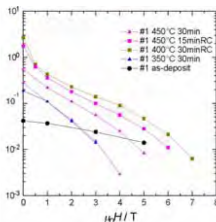
図 75 酸素アニールした Er123/STO の J_c -B カーブ。RC はアニール後急冷を施したことを示す。
