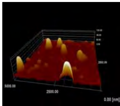
図 41 MOD-Gd123 薄膜表面 AFM 像。
