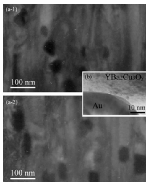
図 68 金を含んだ \text{YBa}_2\text{Cu}_3\text{O}_y 超伝導膜の断面透過電子顕微鏡像
