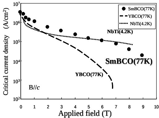
図 17 SmBCO の 77K での J_c 特性
