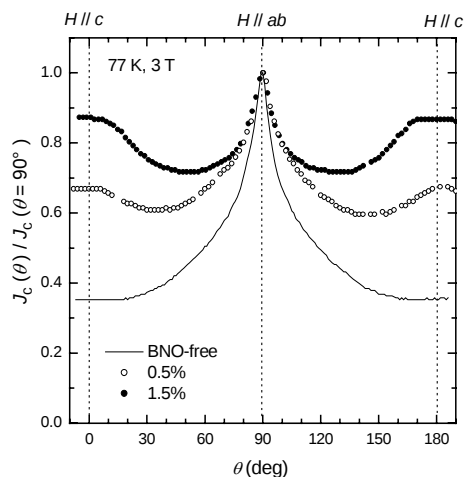
図 83 Er123 および BNO ドープ Er123 薄膜の規格化 J_c の磁場印加角度依存性。
