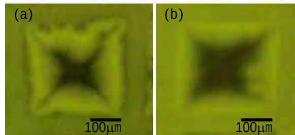
図 72 Er123 薄膜の MO 像。(a)酸素アニール無(b)アニール有
