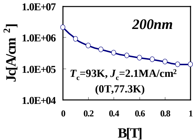
図 47 BaF 2 -Gd123 薄膜の J c 特性
