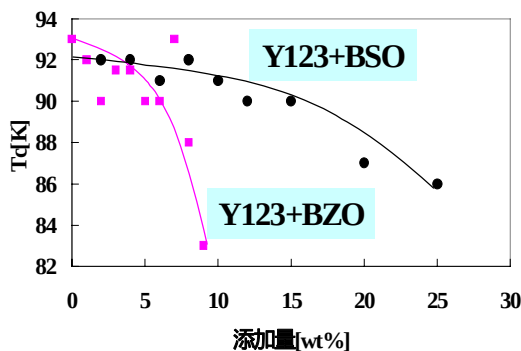
図 52 \text{BaZrO}_3 および \text{BaSnO}_3 添加 Y123 バルク試料における添加量と T_c の関係
