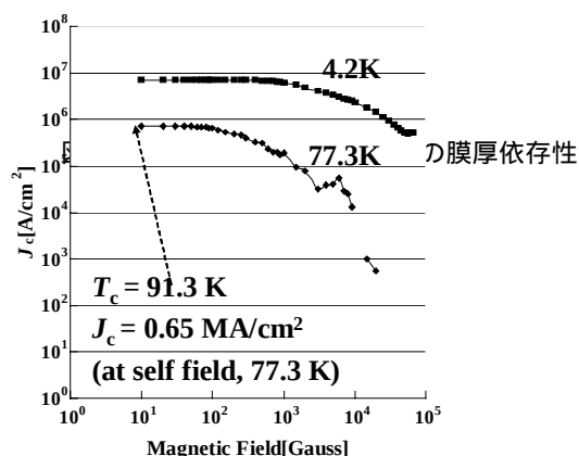
図 43 MOD-Gd123 薄膜の磁場中 J_c 特性。
