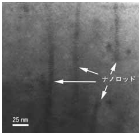
図 56 ナノロッドを含む \text{ErBa}_2\text{Cu}_3\text{O}_y 超伝導膜の断面透過電子顕微鏡像
