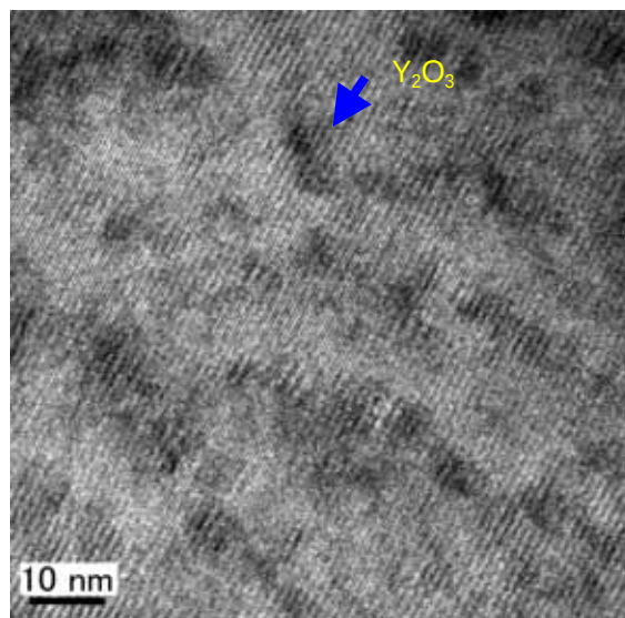
図 69 \text{Y}_2\text{O}_3 を添加した超伝導膜の断面透過電子顕微鏡像
