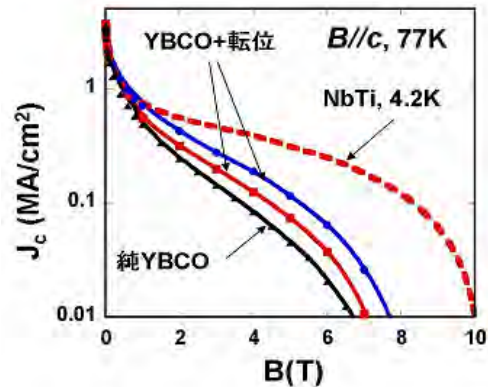
図 10 1 次元 APC を持つ YBCO 薄膜の J_c -B 特性。 \text{Y}_2\text{O}_3 ドープ量と共に J_c が増大する。比較のために 4.2 K における NbTi の J_c -B 特性も示してある。
