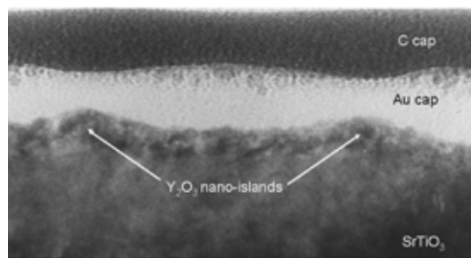
図 54 \text{Y}_2\text{O}_3 ナノアイランドの断面透過電子顕微鏡像
