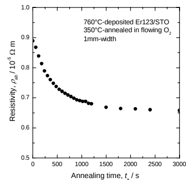
図 73 Er123 薄膜のアニール時間に対する電気抵抗率の変化
