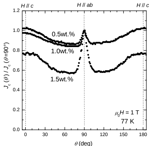
図 82 ささまざまな BZO ドープ量をもつ Er123 薄膜の J_c の角度依存性
