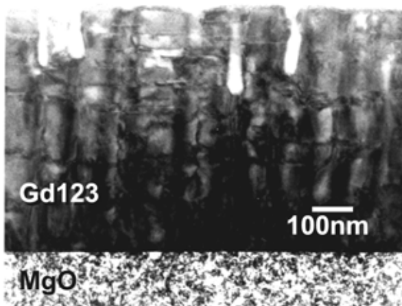
図 64 \text{GdBa}_2\text{Cu}_3\text{O}_y 超伝導膜の断面透過電子顕微鏡像
