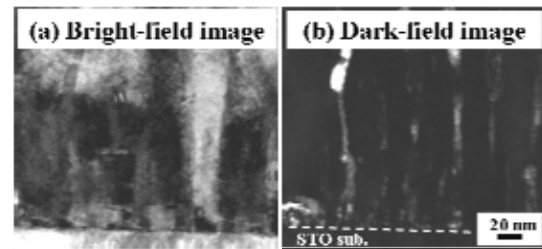
図 36 明視野像(a)および Er123 相以外からの回折斑点で結像した同一視野の暗視野像。
