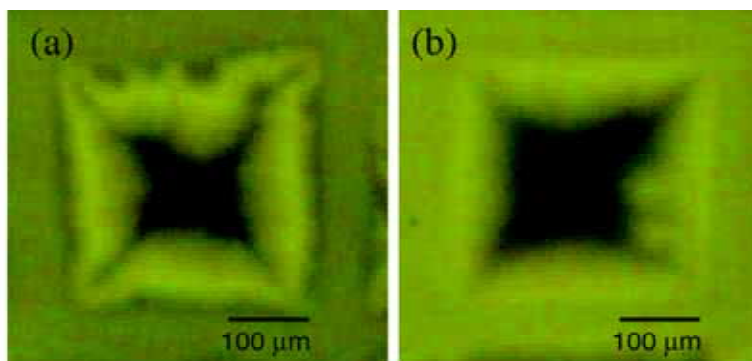
図 70 \text{ErBa}_2\text{Cu}_3\text{O}_y 薄膜の磁気光学像(MOI)。(a)アズデポ膜、(b)酸素アニール後。
