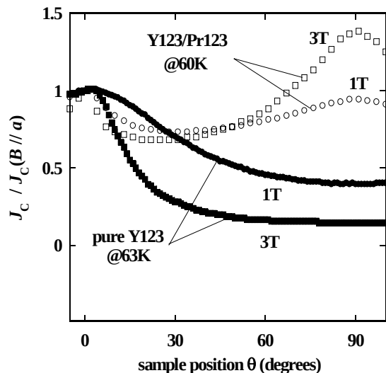
図 26. c -軸方向に絶縁層を層状に導入した a -軸配向膜の 1T と 3T の磁場中での臨界電流密度の磁場角度依存性。
