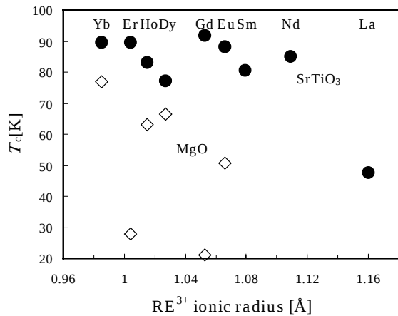
図 38 MOD 薄膜の超伝導転移温度と希土類元素との関係。
