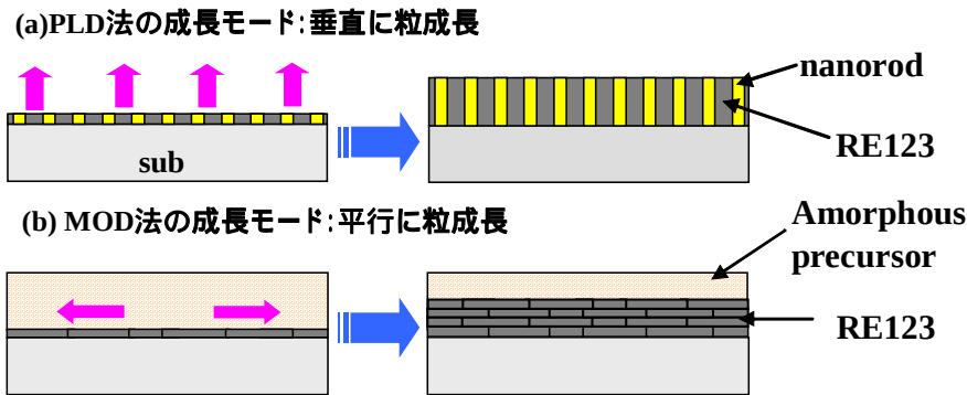
図 37 PLD 法と MOD 法の成長模式図。
