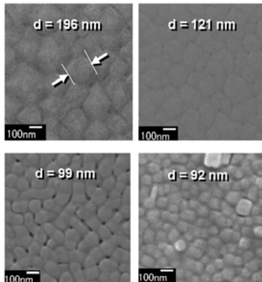
図 12 成膜条件の調整で制御した GdBCO 薄膜の粒径変化。
