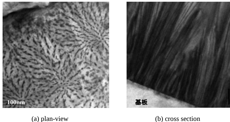
図3 BaZrO 3 ナノロッドを用いた1次元人工ピンの例。(a)ナノロッドを含むY系薄膜を上面観察したもの。細かな粒子状のものがナノロッド。(c)Y系薄膜を横から見たもの。多数のナノロッドが膜面に垂直に成長している。
