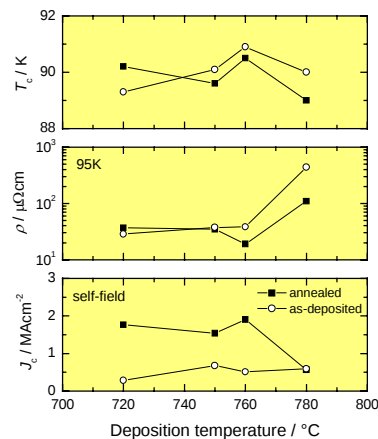
図 71 Er123 薄膜の成膜温度に対する T_c 、電気抵抗率、 J_c の変化
