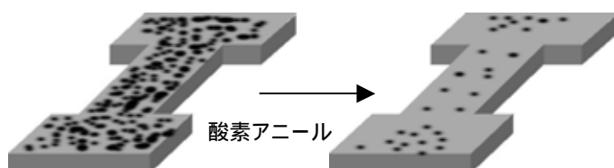
図 74 Er123 薄膜における酸素アニール効果の模式図
