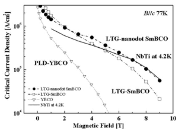
図 21 ナノ析出物を導入した SmBCO 薄膜の J_c -B 特性
