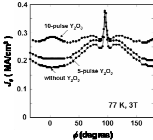
図 11 1 次元 APC を持つ YBCO 薄膜の J_c の磁場印加角度依存性。B//c の J_c が Y_2O_3 量にしたがって増大している。
