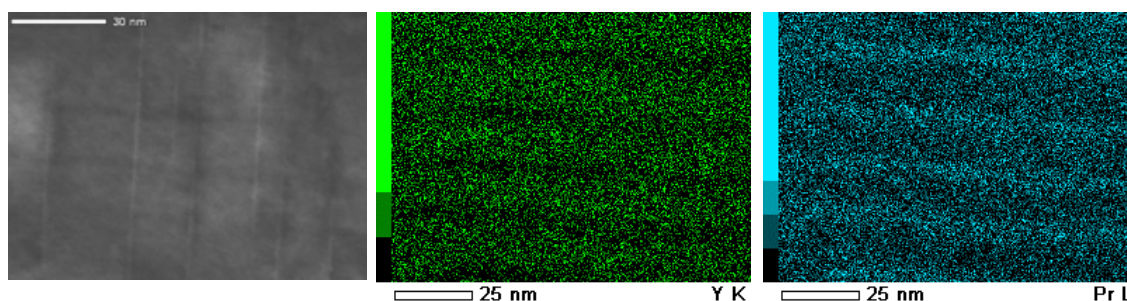
図 67 断面透過電子顕微鏡像とそれに対応する Y、Pr の組成マップ
