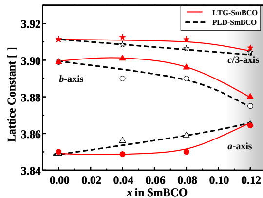
図 19 SmBCO 薄膜の格子定数の変化
