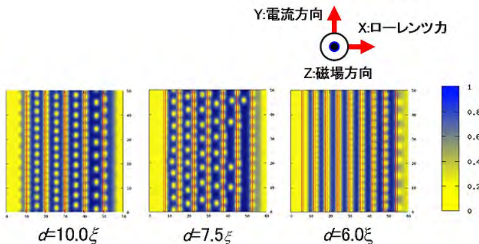
図8 時間依存 GL 方程式に基づいた量子化磁束のピン止めシミュレーション。サイズは 60\xi \times 50\xi で、通電方向に平行なピン止め点が入れてある。d はその間隔。ピン止め点のサイズ、配置によって J_c が大きく異なることが示される。
