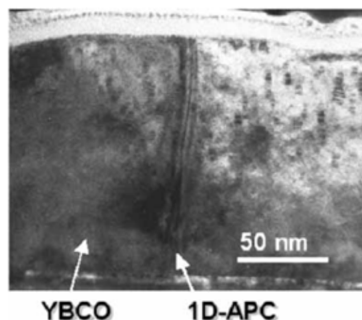
図 55 転位が導入された \text{YBa}_2\text{Cu}_3\text{O}_y 超伝導膜の断面透過電子顕微鏡像
