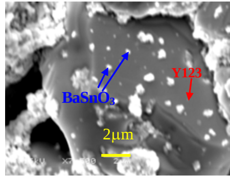
図 51 \text{BaSnO}_3 添加 Y123 試料の SEM 像
