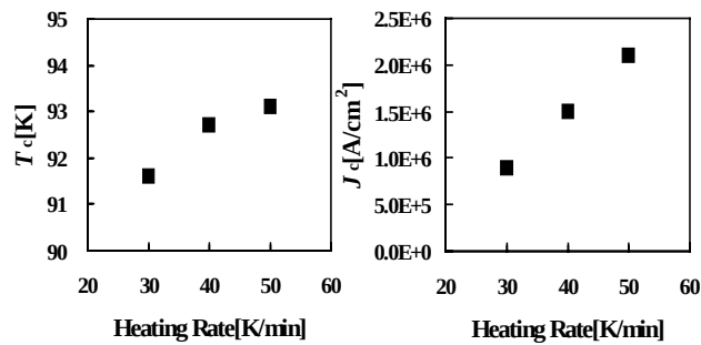
図 45 BaF 2 -Gd123 薄膜の超伝導特性の加熱速度依存性。
