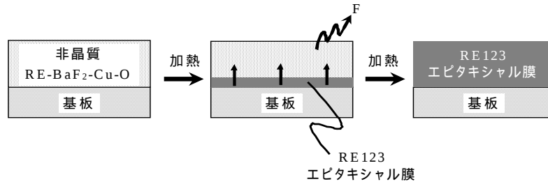
図44 (a)従来のBaF 2 プロセスと(b)本研究で用いた新しいBaF 2 プロセスの模式図。
