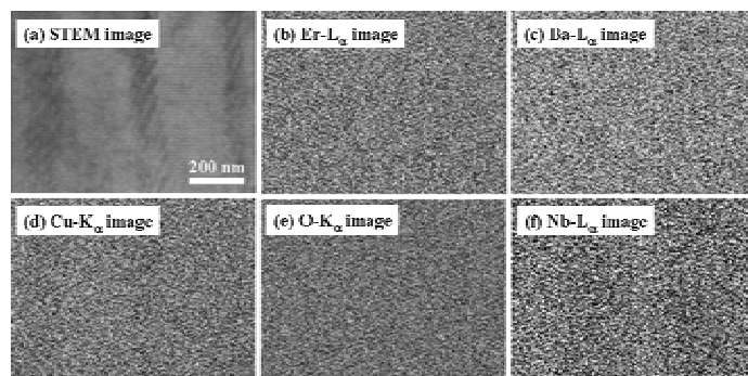
図 33 ナノロッドを含む領域の走査透過電子顕微鏡像(a), および同領域から取得された Er(b), Ba(c), Cu(d), O(e), Nb(f)の特性 X 線像。
