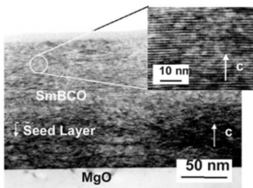
図 15 SmBCO/MgO の断面 TEM 写真
