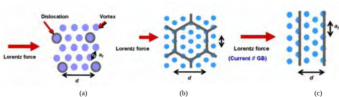
図7 (a) 転位によるピン止め構造、(b)粒界によるピン止め構造、(c)平行粒界によるピン止め構造。
