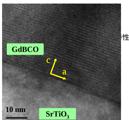
図 42 MOD-Gd123 薄膜断面 TEM 像。
