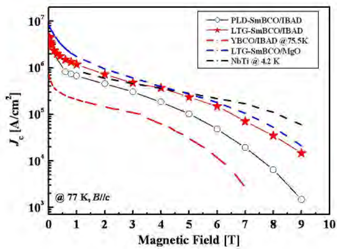
図 89 LTG-SmBCO/IBADが現在のベストデータ。比較のために記した NbTi@4.2 K とほぼ匹敵する値となった。APC 法の有効性を示す結果である。
