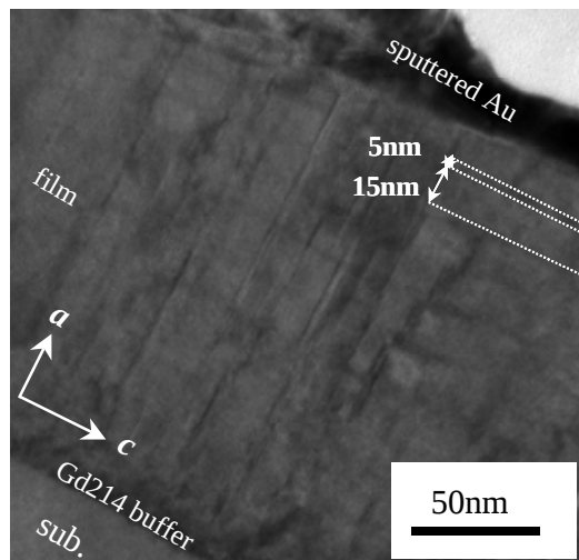
図 25 断面透過電子顕微鏡像。5nm と 15nm の層が交互に積層された a -軸配向膜であると分かった。
