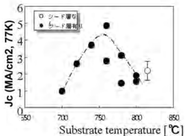
図 16 J_c 特性と基板温度の関係
