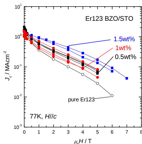
図 81 ささまざまな BZO ドープ量をもつ Er123 薄膜の J_c -B 特性
