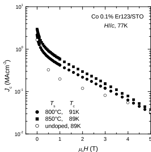
図 80 Co0.1%ドープ Er123 薄膜の J_c -B 特性。
