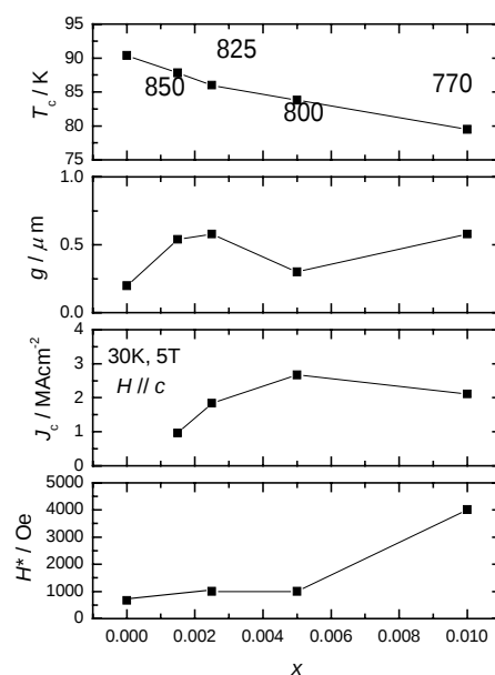
図 76 Co ドープ Er123 薄膜の Co ドープ量に対する T_c 、グレインサイズ、 J_c 、 H^* の変化。
