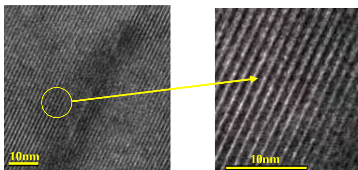
図 49 LaAlO 3 基板上の BaF 2 -Gd 薄膜断面 TEM 像。
