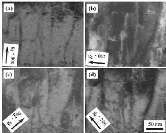
図 30 ナノロッドの縞模様と回折ベクトル ( g_1 \sim g_4 ) との関係を示す明視野像。
