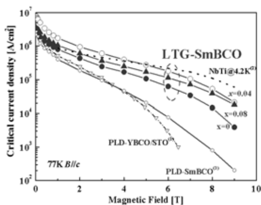
図 20 各種超伝導薄膜の磁場中 J_c 特性の比較
