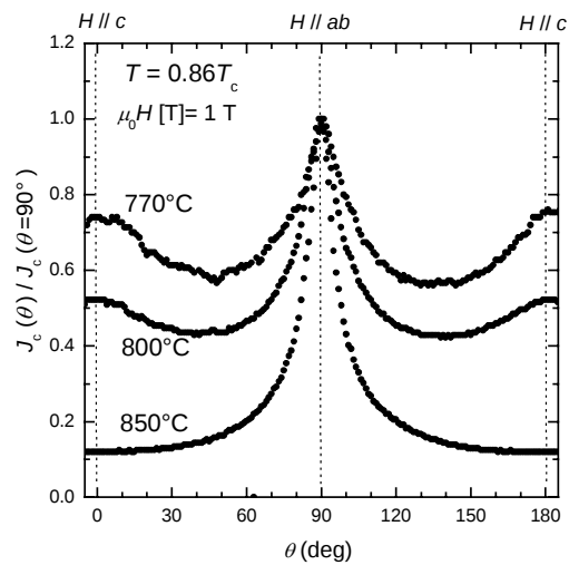
図 77 Co ドープ Er123 薄膜における J_c の角度依存性 (規格化温度 = 0.86T_c )
