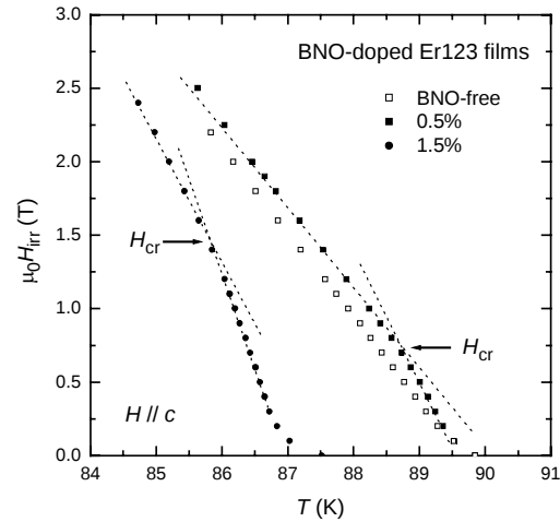
図 85 Er123 および BNO ドープ Er123 薄膜の不可逆曲線。
