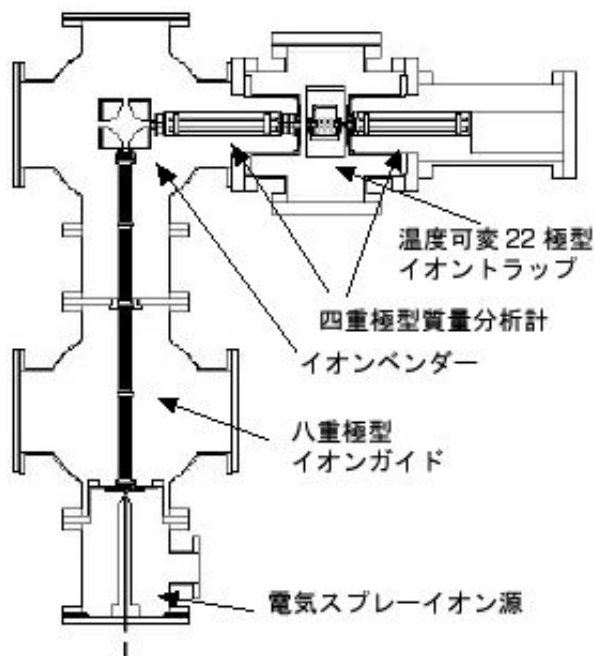
図2 生体分子分光解析装置
