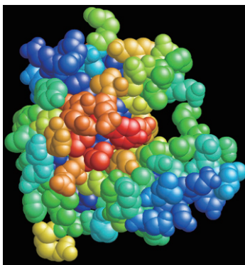
図17: スプライセオゾームの要素タンパク質における推定 RNA 界面
