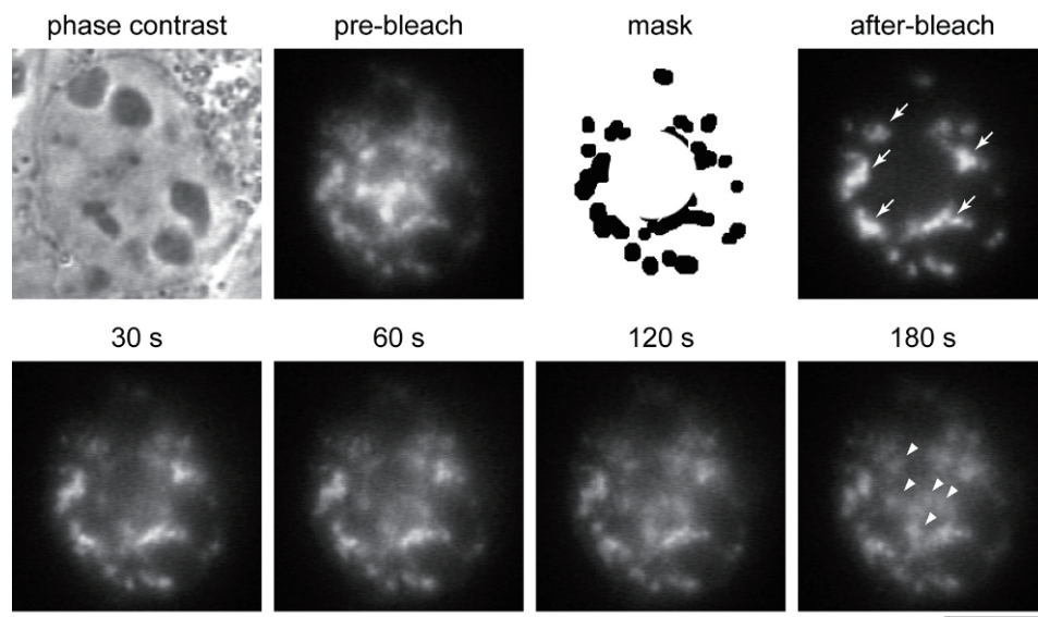
図18 未成熟 mRNA はスペックル間をシャトルする一部のスペックル(矢印)を残して退色させると、退色したスペックルへの mRNA の再結合が見られた。スケールは5 μm
