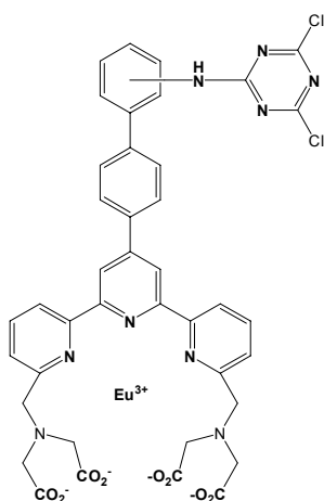
図 1 DTBTA-Eu 3+ の構造
