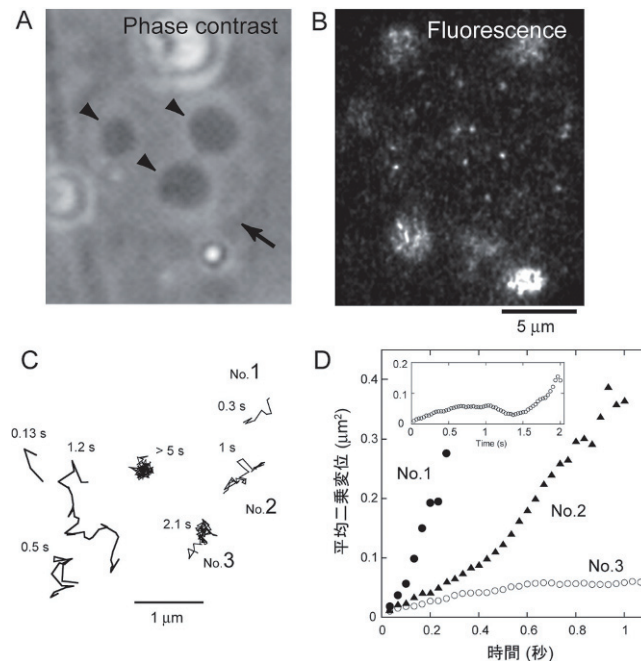
図 15 mRNA の核内運動の軌跡 A6細胞の核内に \beta -globin の mRNA をマイクロインジェクションし、運動を観察した。(A) 位相差像。矢印は核、矢じりは核小体を示す。(B) 蛍光顕微鏡ビデオ像。小さい輝点が 1 分子の mRNA である。周囲の大きな明るい塊は細胞の自家蛍光である。(C) 代表的な mRNA 分子の軌跡。観察時間を左上に示した。(D) C の No.1、No.2、No.3 分子の平均二乗変位を時間に対してプロットした図。挿入図は No.3 の分子を 2 秒間観察したもの。
