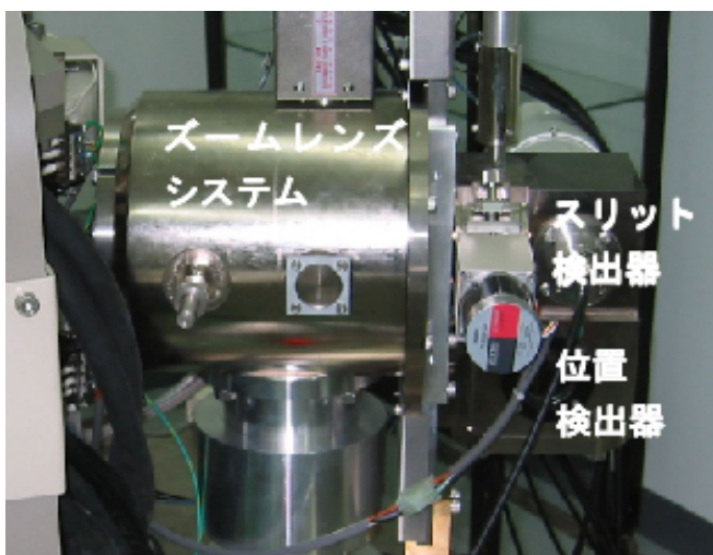
図 10 検出器部分の外観
