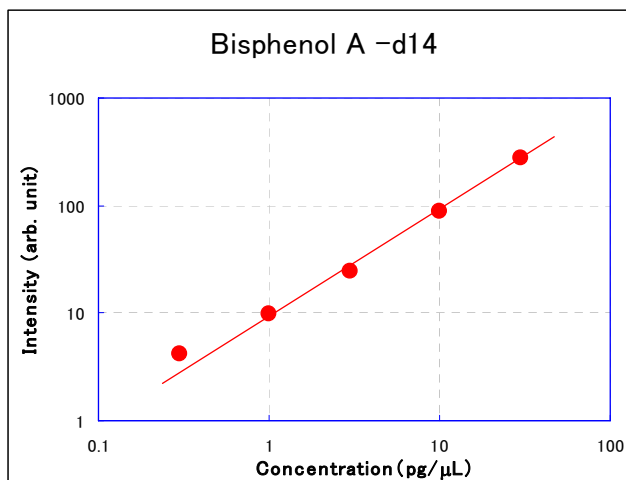
図 1 5 ビスフェノール A-d14 の校正曲線
