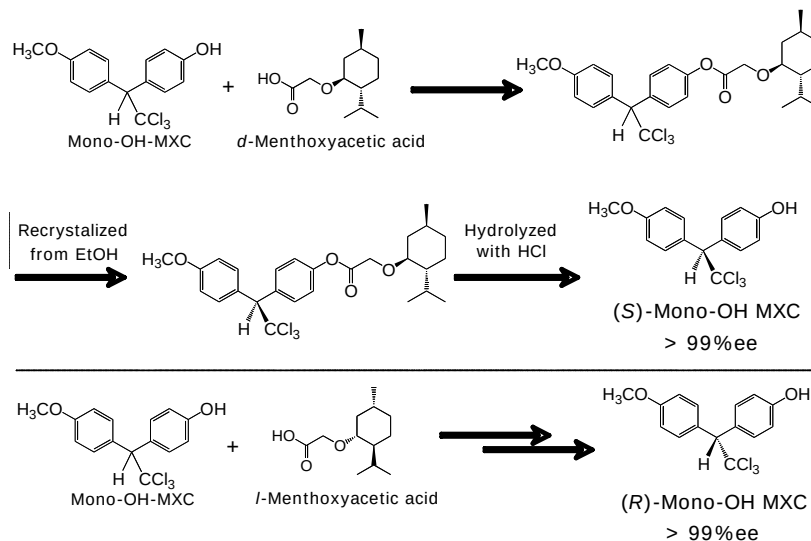
図 6. Mono-OH-MXC の光学分割
