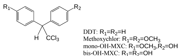
図 1. DDT およびメトキシクロルとその代謝物の構造
