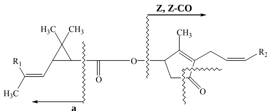
図1 ピレスロイドの一般的開裂様式
