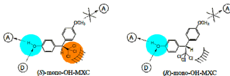
図 14 Mono-OH-MXC の光学異性体とエストロゲン受容体の推定相互作用モデル
