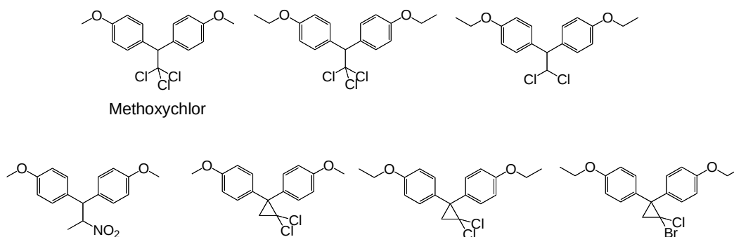
図 4. 代謝反応後にエストロゲン受容体結合活性の増大を示した化合物
