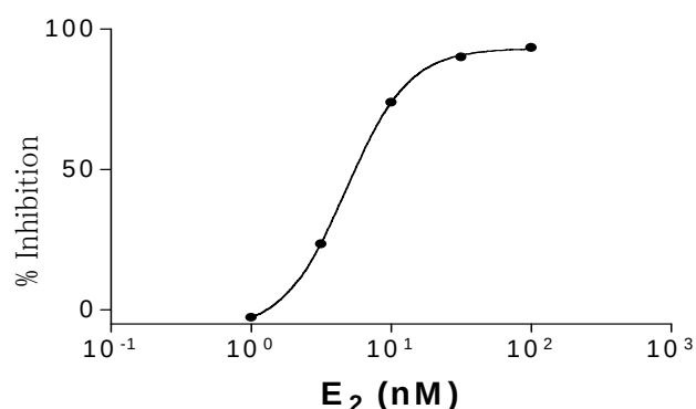
図 10. E 2 による抗 E 2 抗体と E 2 -BSA 結合体との結合阻害
