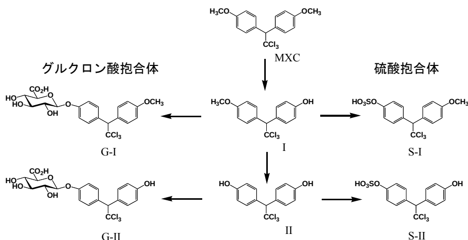
図 7. メトキシクロルの第 I 相および第 II 相代謝反応生成物
