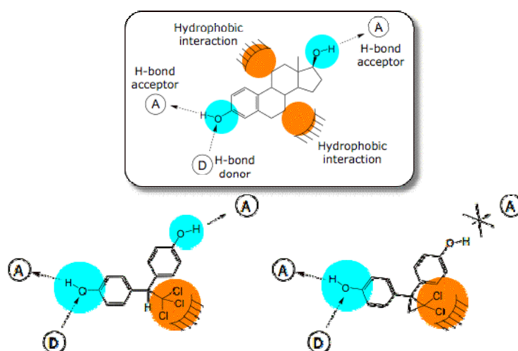
図 13 エストロゲン受容体と DDT 類縁体の推定相互作用モデル
