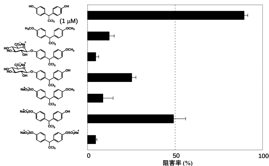
図 8. メトキシクロル第Ⅱ相代謝反応物のエストロゲン受容体結合活性（メトキシクロルは 1μM, それ以外は 10μM の濃度で測定）
