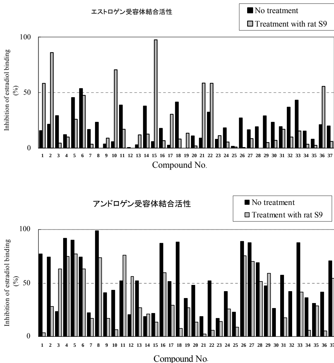
図 3. DDT 類縁体およびその代謝混合物のエストロゲンならびにアンドロゲン受容体結合活性 (測定濃度=38 \mu M)
