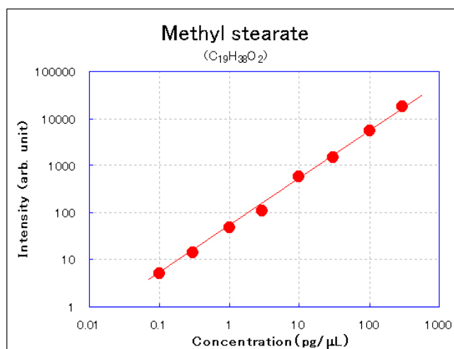
図 1 4 ステアリン酸メチルの較正曲線。
