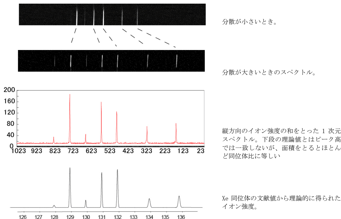
図 1 3 Xe の 2 次元スペクトル。
