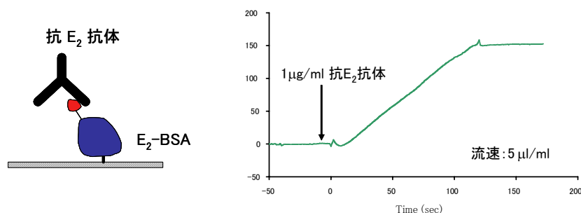
図 9. SPR センサーによる E_2 -BSA 結合体と抗 E_2 抗体との結合の測定
