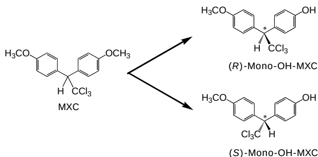
図 5. メトキシクロルおよび mono-OH-MTX の構造
