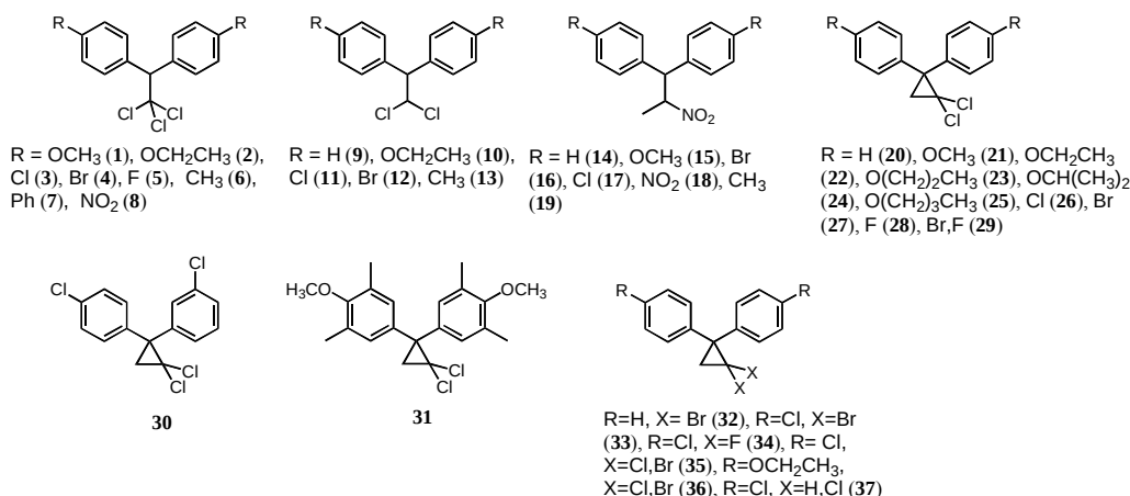
図 2. 活性測定に用いた DDT 類縁体の構造
