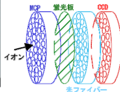
図 11 2次元位置検出器の模式図
