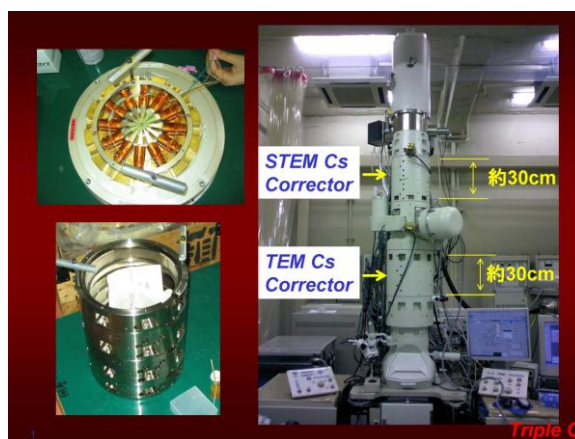
図 2. 一号試作機 Cs コレクタ部(左)と装置外観(右)
