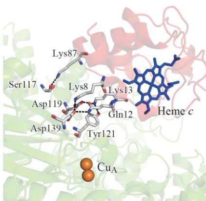
図11. チトクロム c とチトクロム c 酸化酵素の相互作用
