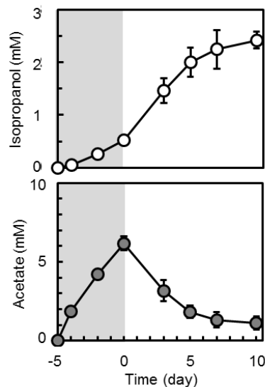
図 3-1,2 イソプロパノール生産 図中灰色部分は暗・嫌気条件、白色部分は光合成条件を示す。
