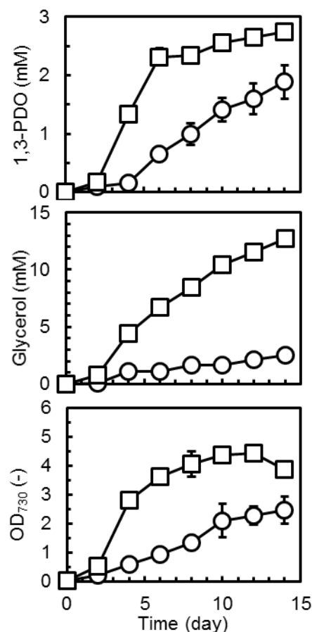
図 3-1,3 1,3-PDO 生産 ○ : 0.04% CO 2 通気、□ : 1% CO 2 通気
