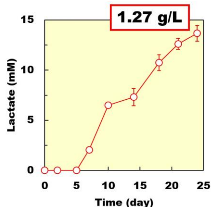
図 3-1,5 乳酸生産
