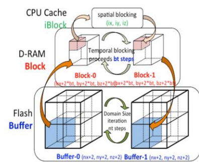
図 C-1 L3-Cache, DRAM, FlashSSD 多階層利用 時間・空間ブロッキングによるステンシル計算
