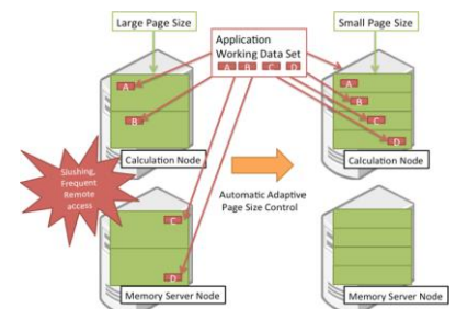
図 C-8 ページサイズ変更とスラッシング回避の原理
