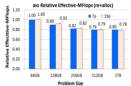
図 C-6 aio 手法（NUMA）ステンシル計算
