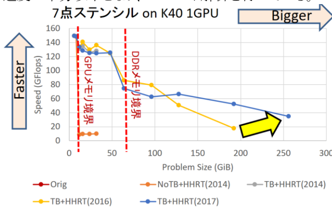
図 A-2: HHRT を用いたステンシル計算の問題規模と性能
