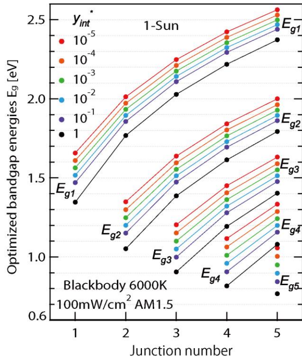
図 13. 多接合太陽電池のエネルギー変換効率と最適バンドギャップエネルギー
