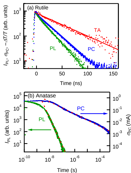
図 1. (a) ルチル型構造における PL, PC, TA の減数曲線。ナノ秒の指数関数減衰を示す。(b) アナターゼ型の非指数関数的な減衰。
