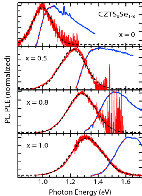
図4. \text{Cu}_2\text{ZnSn}(\text{S}_x\text{Se}_{1-x})_4 単結晶の発光および発光スペクトル。
