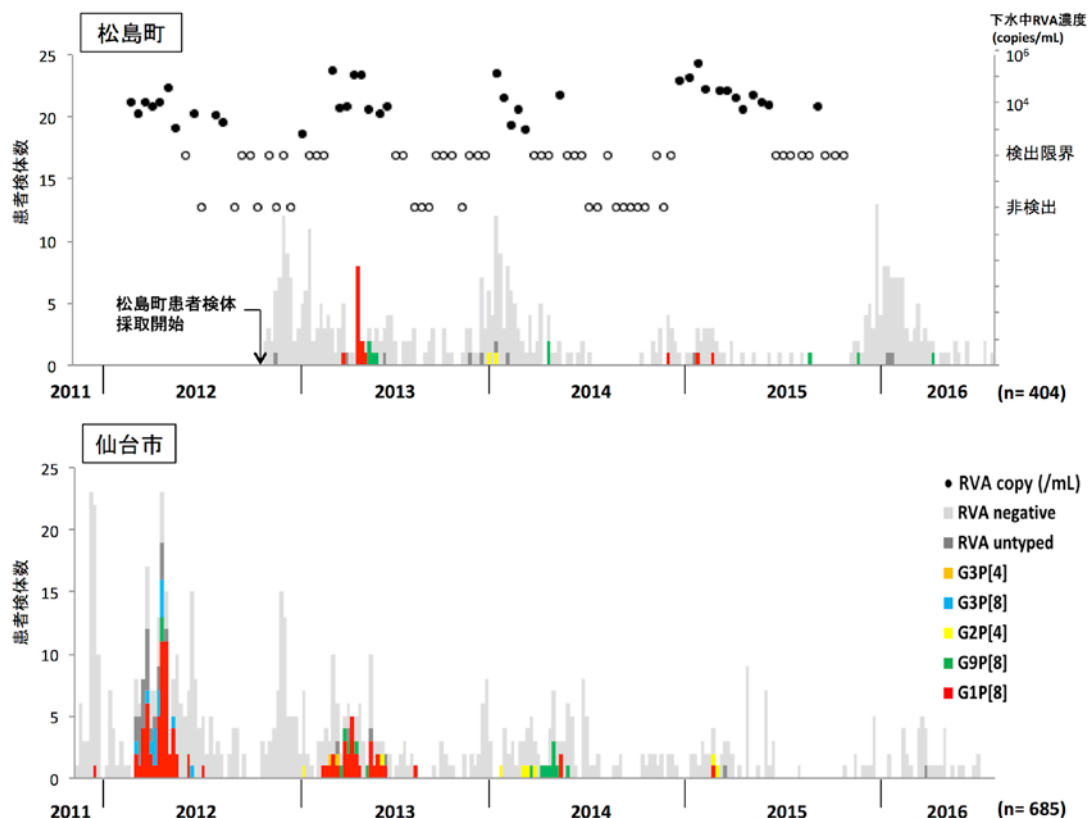
図 4-3. ワクチン導入後、松島町及び仙台市で得られた急性胃腸炎患者検体から検出されたロタウイルス(RVA)の経時的变化と、同時期に松島町で採取された下水試料中の RVA 濃度の経時的变化
