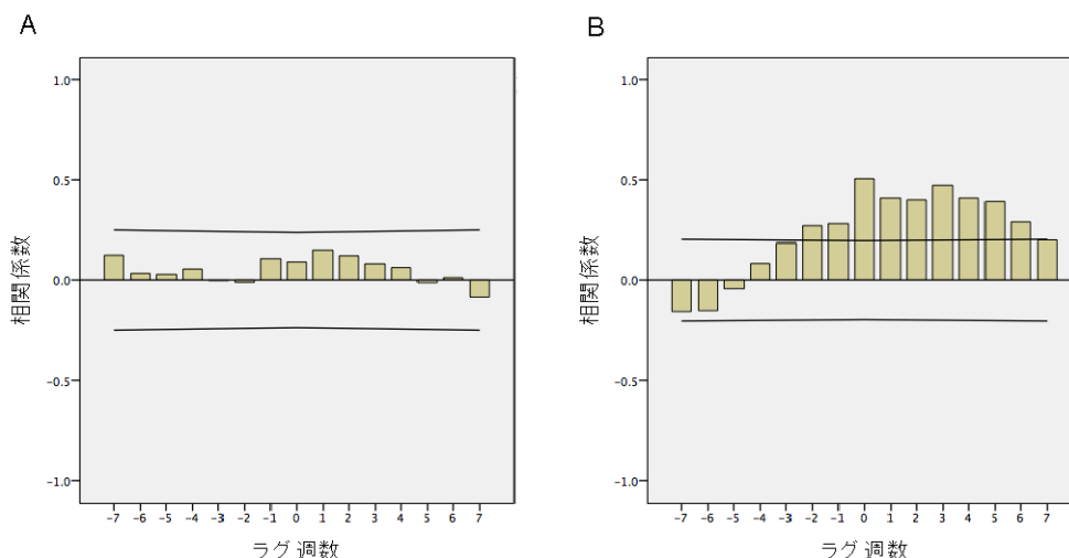
図 1-3. 胃腸炎患者報告数に対する下水中ノロウイルス濃度の相互相関分析結果。A: ノロウイルスGI濃度, B: ノロウイルスGII濃度。図中の横線は、「患者報告数と下水中ノロウイルス濃度が相関しない」という仮説が、5%の確率で成立する範囲を示す。
