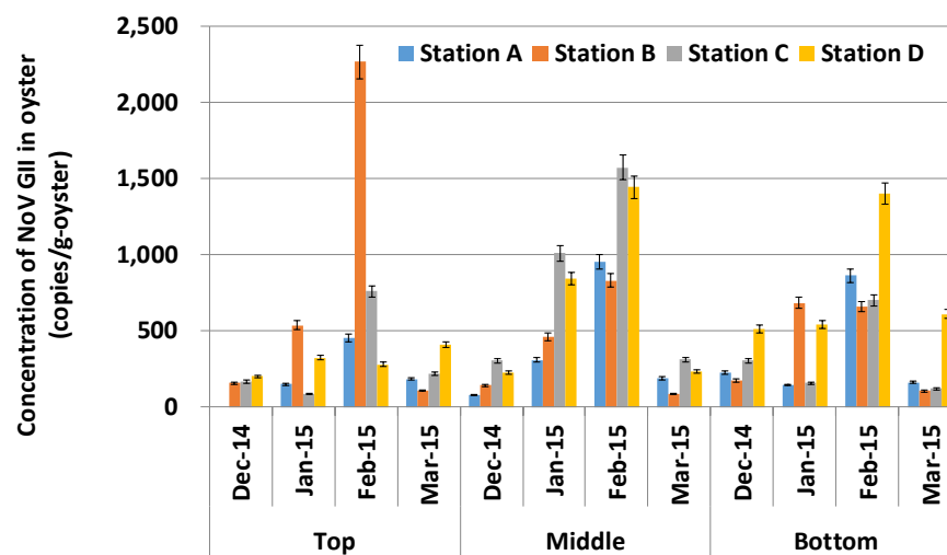
図 2-3. 地点・深度・月別のカキに含まれるノロウイルス量(2014-2015 年シーズン)
