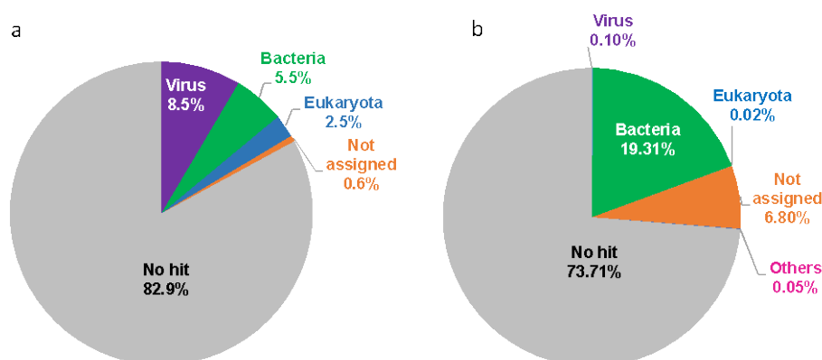
図 1-1. 下水試料のメタゲノム解析で得られた配列の分類と配列数の割合。ポリ A 鎖を有する RNA を特異的に回収する技術を適用した結果を a, 適用しなかった結果を b に示す。
