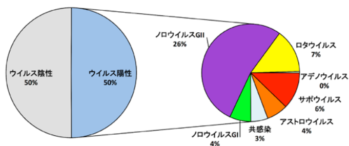
図 4-1. 急性感染性胃腸炎患者から検出されたウイルスの推移(上図, 2012 年 11 月 -2016 年 7 月, 松島町)及び、その内訳(左図)
