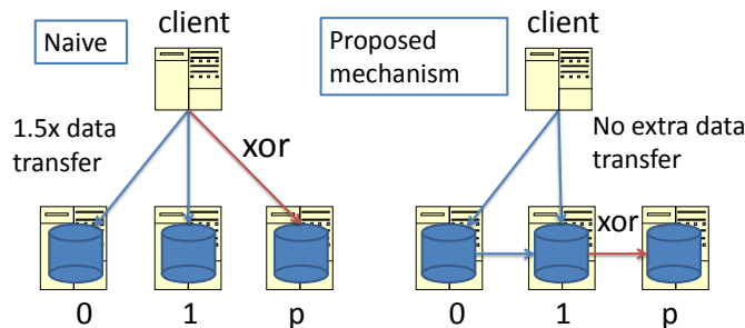
図 2. 2D1P の RAID-4 のアクティブストレージによるデータ転送と冗長コード計算
