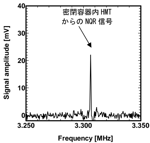
図6 NQR スペクトル
