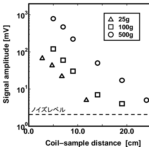
図8 NQR 信号の HMT 重量依存性
