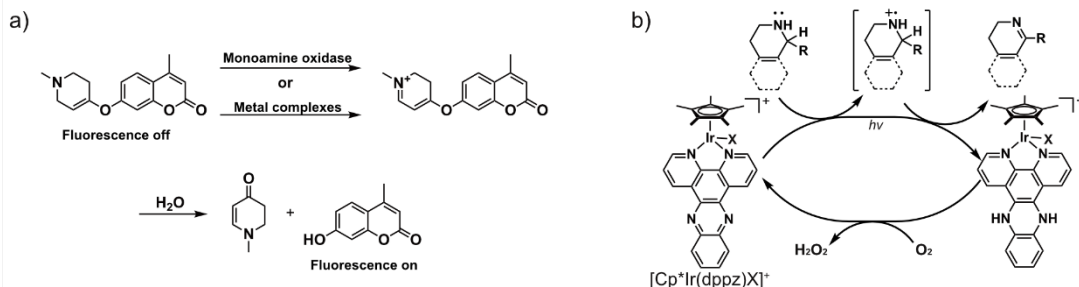
図 1. (a) 合成錯体のスクリーニングのための turn-on 型蛍光基質、(b) [\text{Cp}^*\text{Ir}(\text{dppz})\text{Cl}]^+ による含窒素化合物の脱水素化の反応機構
