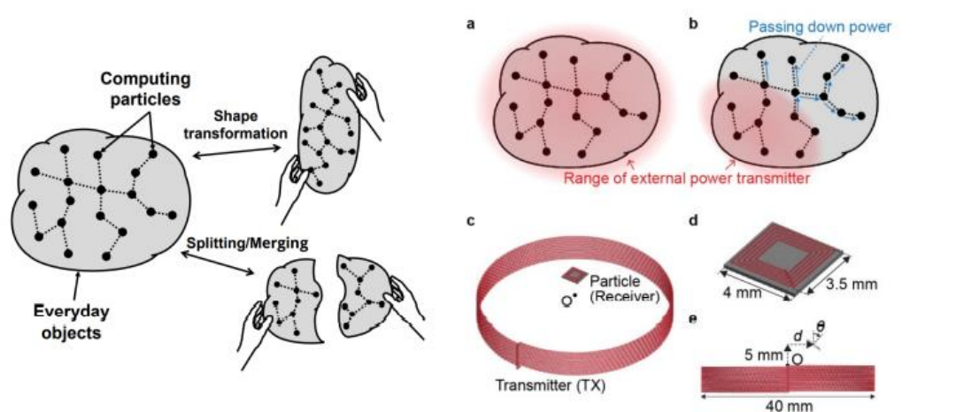
図 2 形状変化するコンピュータの無線ネットワーキングに向けた給電技術の検討。(a) 全体に対して送電器から電力を供給する方法と、(b) 一部の粒子にのみ電力を供給し、粒子間のネットワークにより電力を送り届ける方法。(c, d) 電磁界解析による粒子状のコンピュータへの無線電力伝送技術の検討。
