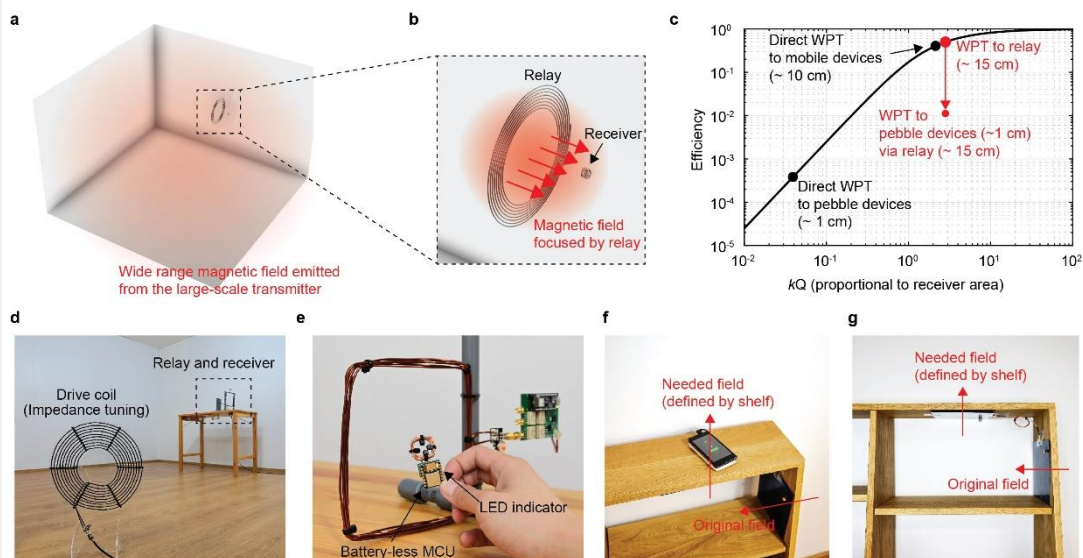
図 1 小型機器への広範囲な給電に向けた階層的な共振器。(c) 階層性により高効率となる要因の解析。(d) 実験時の部屋スケールマルチモード準静空洞共振器の中の様子。(e) 磁界の集中による小型マイコンへの給電。(f, g) 磁界を曲げることによる棚の上のモバイル機器への給電。
