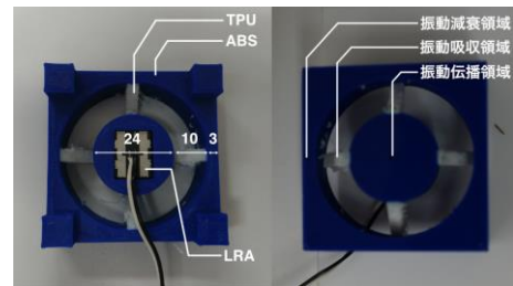
図 3: 振動子と振動伝播/吸収構造
