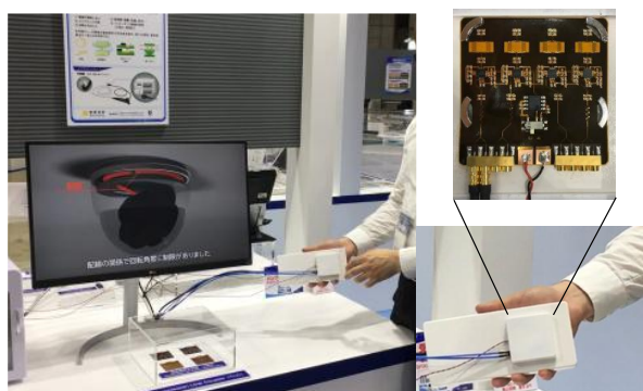
図2.1.3 TLC非接触コネクタによる高精細画像伝送デモ
