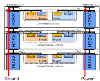
図 1.1.2 HDSV 技術
