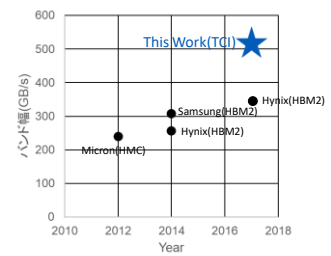
図 1.1.1 達成した TCI 積層 DRAM の性能
