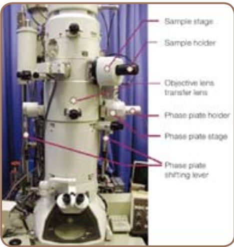
Phase-contrast TEM
