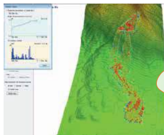
アラナヤケ地すべり発生時の 降雨と土砂流動の再現
