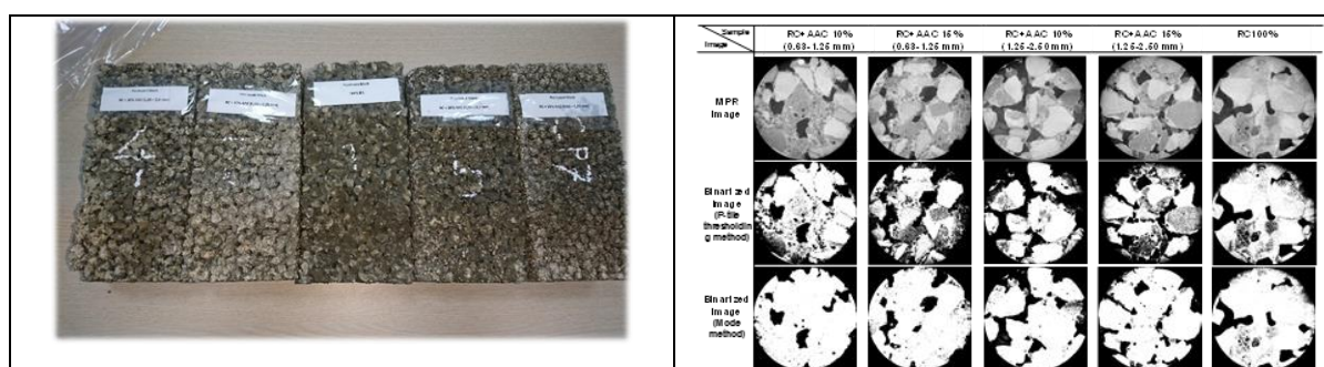
図4 ベトナム建廃リサイクル材を用いた透水性舗装ブロック：左）顆粒状軽量気泡コンクリート材の混合比率を変化させて作成したブロック材、右）マイクロフォーカス X 線 CT 装置を用いた間隙構造解析
