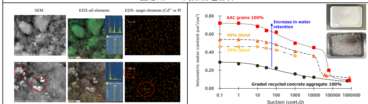
図5 技術開発研究例。左：顆粒状軽量気泡コンクリート材による水中重金属除去能評価、右：顆粒状軽量気泡コンクリート材混入路盤材の保水性評価
