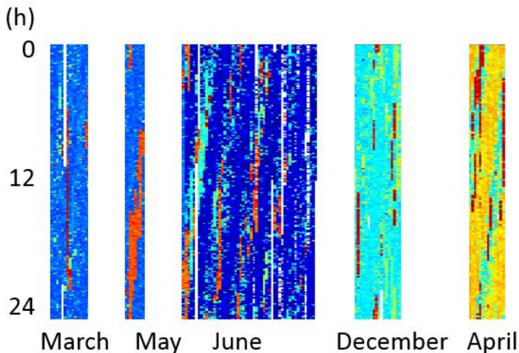
図6 LIDOで2016年に記録した水中音の季節変化。機械学習で分類された音種は季節によって異なっ
