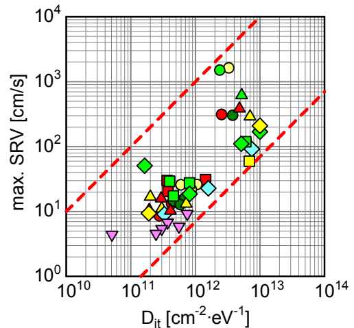
Fig.1-1 各種パッシベーション膜の界面トラップ密度と再結合速度の関係
