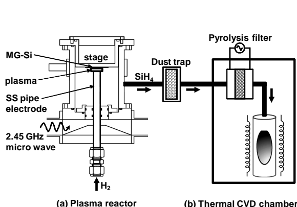
図 1 金属級 Si 原料から生成した SiH 4 ガスを用いた熱 CVD プロセス
