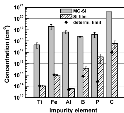
図 2 金属級 Si および本方法により形成した Si 中の不純物濃度
