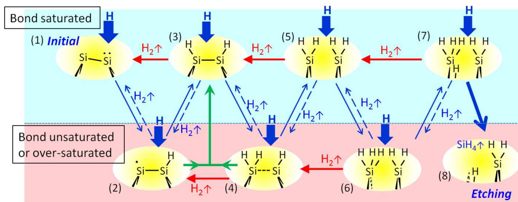
図3 HラジカルによるSiエッチングの素過程
