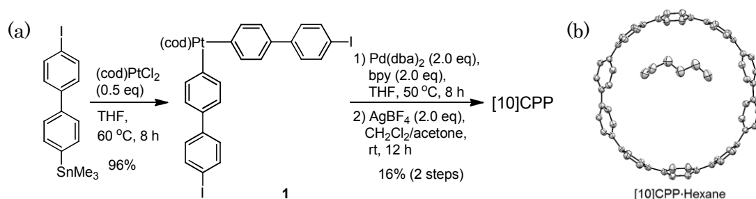
図 2. (a) シスビアリアル白金錯体 1 を経る選択的[10]CPP 合成法と、(b)単結晶 X 線構造解析により得られた[10]CPP の構造
