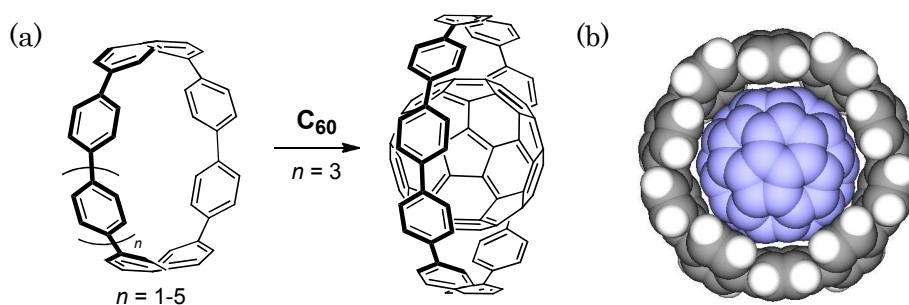
図 1. (a) [10]CPP による C 60 のサイズ選択的な包接と (b) 包摂体の CPK モデル
