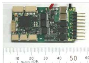
D-RMTPIII搭載小型分散モータドライバ(駆動部・制御部分離)
