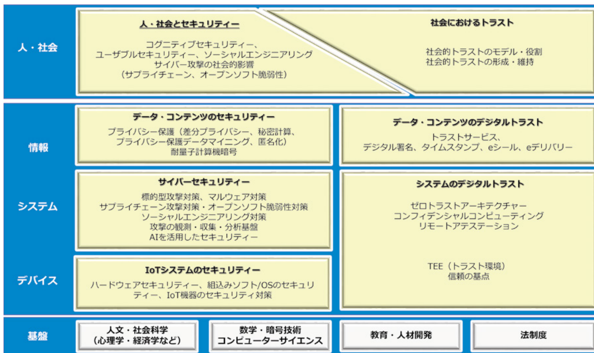
図 2-4-2 セキュリティー・トラストの俯瞰図 (構造)
