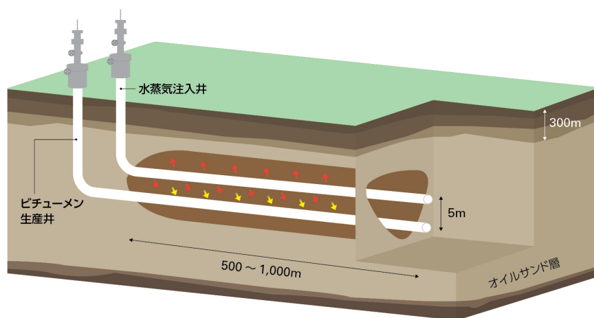
図2.1-1 カナダのSAGD法による重質油の生産概略図
