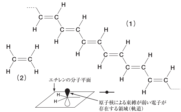
図1 エチレンの炭素原子が持つ電子の軌道とその軌道に電子が入っている様子を示す図
