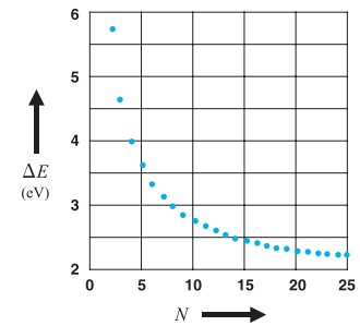
図5 エチレン単位数 N とエネルギー差 \Delta E との関係
