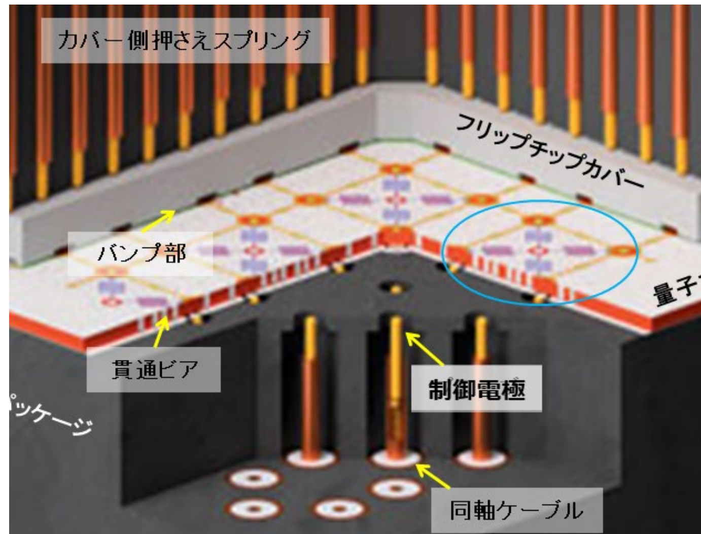
量子ビット基板の3次元実装方式
