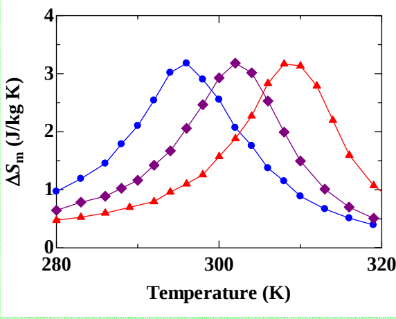
図3 キュリー温度 T_c を異なる値に制御した球状材料の磁気エントロピー変化 \Delta S_m の温度変化。
