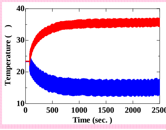
図4 水素化球状材料を用いた熱分離試験結果。温度差20を実証。
