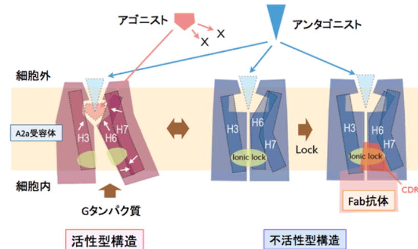
図3. 抗体を用いて創薬標的膜たんぱく質の結晶構造を得ることに成功
