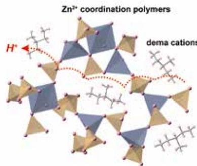
図3 配位高分子ガラスの3次元ネットワーク イメージ図
