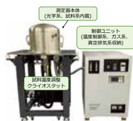
図1 商品化熱膨張計システムの外観 光学系、試料系はチャンバー内に内蔵されている。制御ユニット内には、温度制御系、ガス系、真空排気系が収納。
