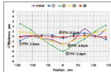
図3 TTV自動補正による300mmTSVウェーハ研削時のTTV食い込み結果。
