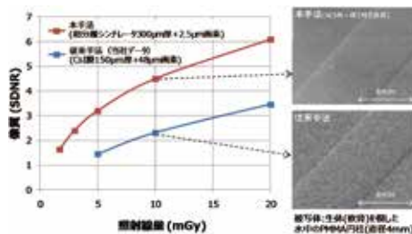
照射線量と像質の関係(左)と、X線位相コントラスト像(右)
