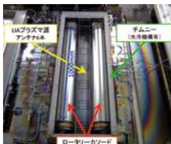
デュアル・ロータリーカソード型LIAスパッタ源
