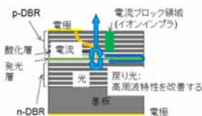
横方向結合共振器を導入した面発光レーザ断面図
