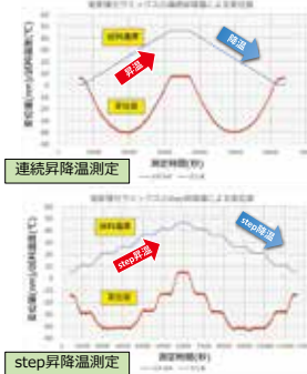
図2 低膨張セラミックスの試料温度に対する変位量(連続昇降温測定とステップ昇降温測定の比較)
