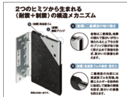
DIT制振筋かい金物の構造メカニズム
