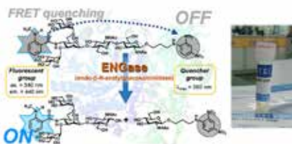
FRET消光解消を作用原理としたENGaseの活性検出
