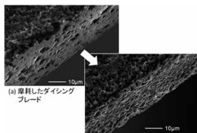
放電ドレッシング前後のダイシングブレード面
