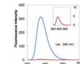
MM3Dおよび加水分解物の蛍光スペクトル
