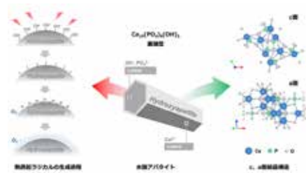
図2 HAp表面における熱励起ラジカル生成過程
