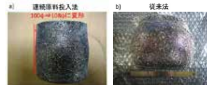
(a)原料連続投入法によるリチャージ6回育成後のルツボと (b)従来法によるリチャージ6回育成後のルツボの写真
