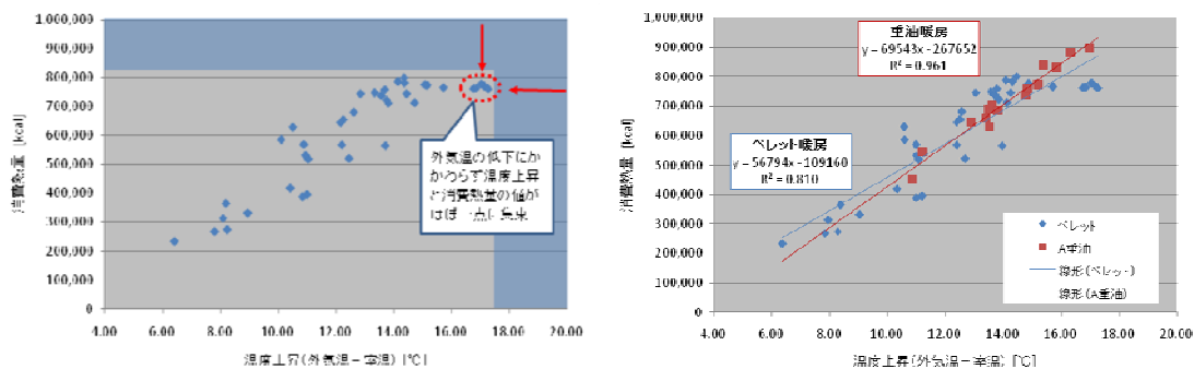
図 3-2. 加温実証試験におけるシステムの比較調査結果(2007 年度) (左: ペレット暖房による室温の上昇と消費熱量の関係、右ペレット暖房システムと重油暖房システムのエネルギー効率比較)
