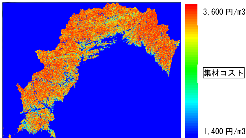
図 3-10. 集材コスト分布図
