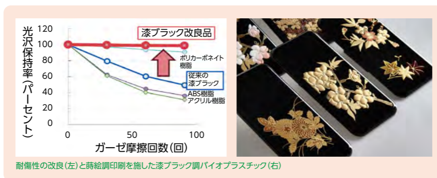
耐傷性の改良(左)と蒔絵調印刷を施した漆ブラック調バイオプラスチック(右)
