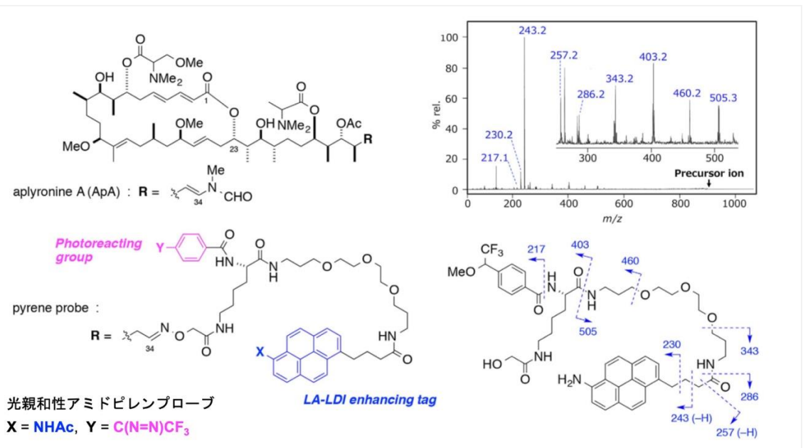
図1 アプリロニン A の光親和性アミドピレンプローブの構造と LA-LDI MS/MS 解析
