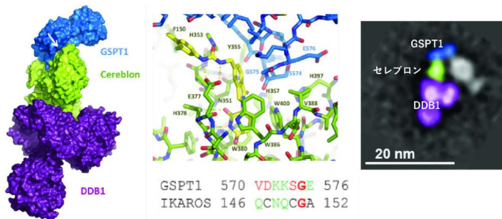
図1 セレブロン(Cereblon)と CC-885, GSPT1 との結合の構造基盤。
