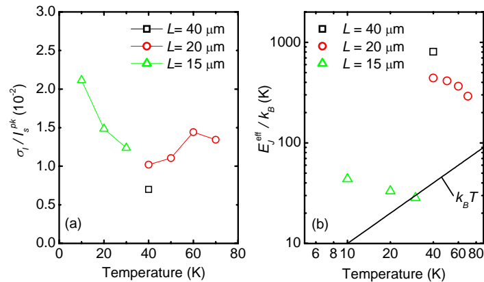
図 3 (a) スwitching 電流分布幅の温度依存性 (b) 実効的ジョセフソンエネルギーの温度依存性
