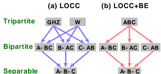
図 2. (a) LOCC と (b) 束縛エンタングルメント (BE) を利用した LOCC における 3 量子ビットの純粋状態の分類と変換性。
