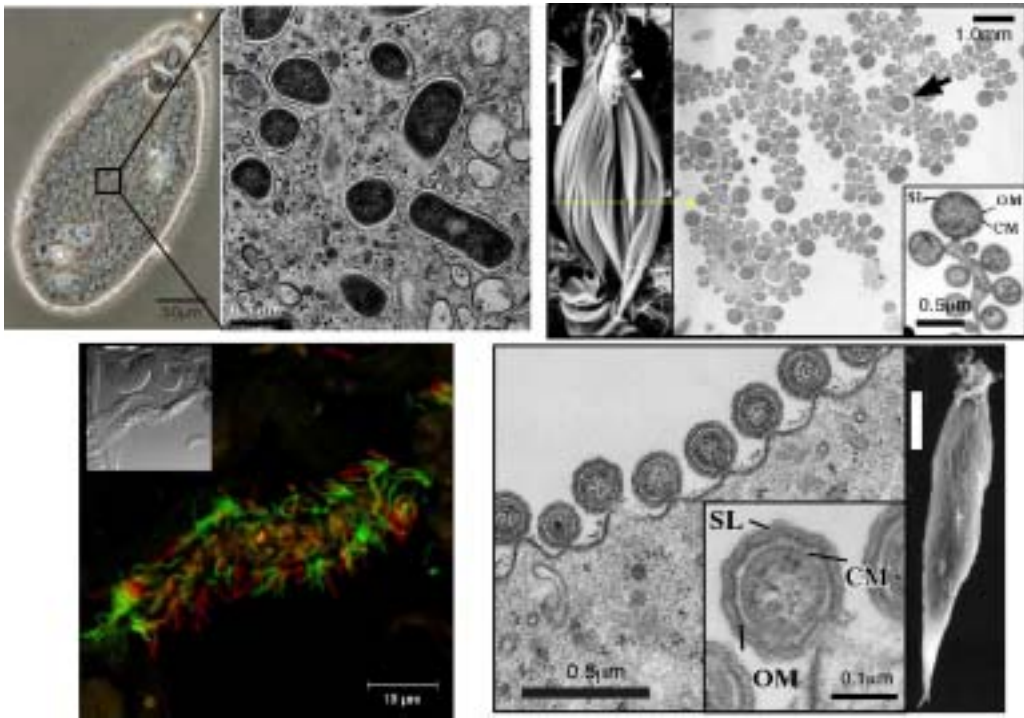
左上、原生生物 Eucomonympha sp. と細胞内共生スピロヘータの TEM 像。左下、 Dinenumpha porteri の細胞表層に共生する 2 種のスピロヘータの FISH。右上、 Hoplonympha sp. の SEM 像 (scale, 10 \mu\text{m} ) と細胞表層に共生する Bacteroidales 細菌の TEM 像。矢印は細胞内に取り込まれた細菌細胞。右下、 Devescovina sp. の SEM 像 (scale, 10 \mu\text{m} ) と細胞表層に共生する Bacteroidales 細菌の TEM 像。SL, surface layer; OM, outer membrane; CM, Cellular membrane。
