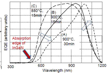
図 C-10. n-InGaN 成長直前の AlN/Si 基板の NH 3 気流中熱処理条件の異なる n-InGaN/AlN/pn-Si 構造の分光感度特性
