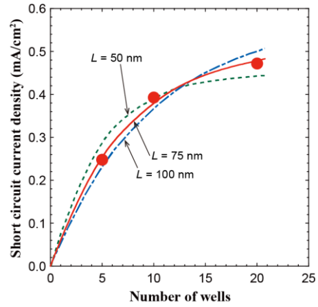
図 B-2. InGaIn/GaN MQW 太陽電池における短絡電流の井戸数依存性。曲線はいくつかの特性長に対する式(1)による計算値。
