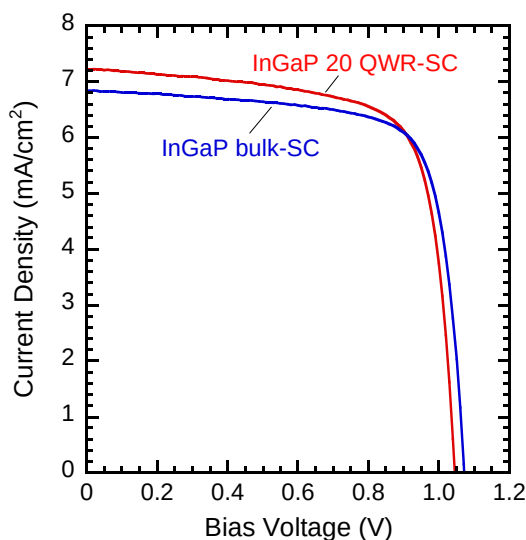
図 B-8. 傾斜角 10^\circ の基板上に成長した量子細線構造 (QWR) 及び InGaP バルク層を光吸収層とする単体セルの電流－電圧特性
