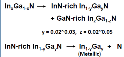
図 C-12. 成長温度 650^\circ\text{C} 付近での \text{In}_x\text{Ga}_{1-x}\text{N} の相分離のスキーム
