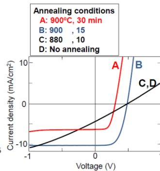
図 C-9. n-InGaN 成長直前の AlN/Si 基板の NH 3 気流中熱処理条件の異なる n-InGaN/AlN/pn-Si 構造の発電特性
