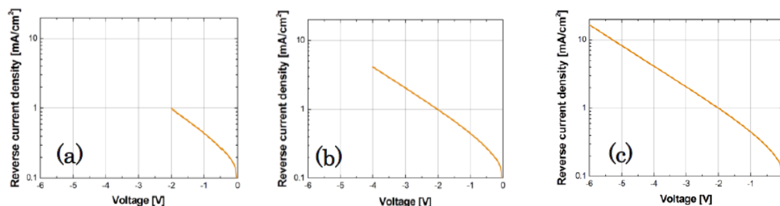
図 A-8. 300 秒照射後の p\text{-Si}/n\text{-Si} 接合の逆方向の電流-電圧特性。(a) : 0 V \rightarrow -2 V \rightarrow 0 V。 (b) : 0 V \rightarrow -4 V \rightarrow 0 V。(c) : 0 V \rightarrow -8 V \rightarrow 0 V。
