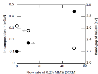
図 C-20. 異なる MMSi 流量で成長させた InGaN 膜の In 組成と禁止帯幅
