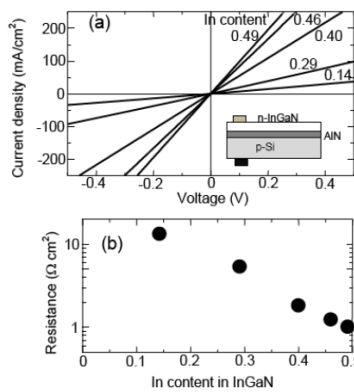
図 C-8. In 組成 0.1~0.5 の n-InGaN を成長させた n-InGaN/AlN/p-Si 構造の電気伝導特性
