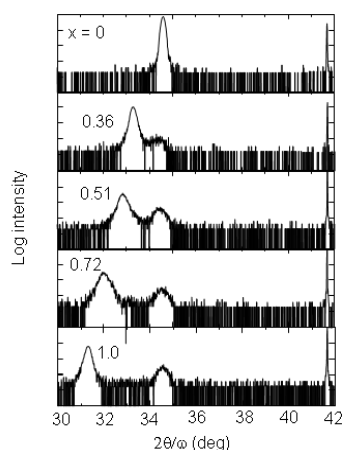
図 C-2. サファイア(0001)基板上に GaN バッファ層を用いて成長させた In_xGa_{1-x}N ( x = 0 \sim 1 ) の X 線 2\theta/\omega 回折図形。
