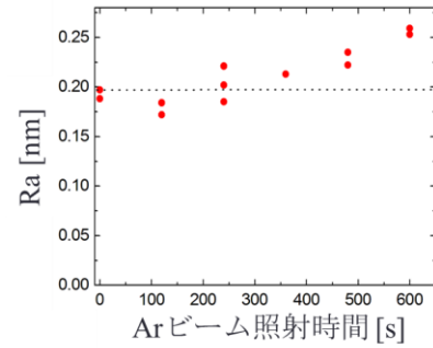
図 A-4. Si 基板表面の Ra の Ar ビーム照射時間依存性。
