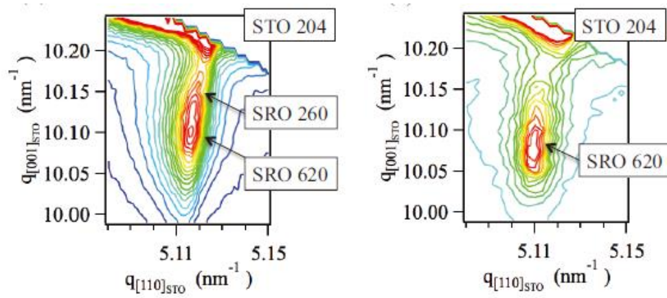
図 3-6 SrRuO 3 ナノワイヤーの局所逆格子マップ。 左は0.2 × 0.2 mm 2 のビームで、右は250 × 190 nm 2 のビームで測定。左ではツイン構造に起因する260回折と620回折が観測されているが、右では620回折のみが観測された。
