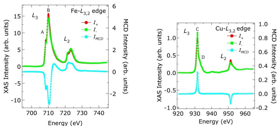
図 3-2 \text{CaCu}_3\text{Fe}_4\text{O}_{12} のFe-L、およびCu-L吸収端でのXAS・XMCDスペクトル
