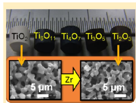
図 2-3 多孔質Ti n O 2n-1 モノリスの作製
