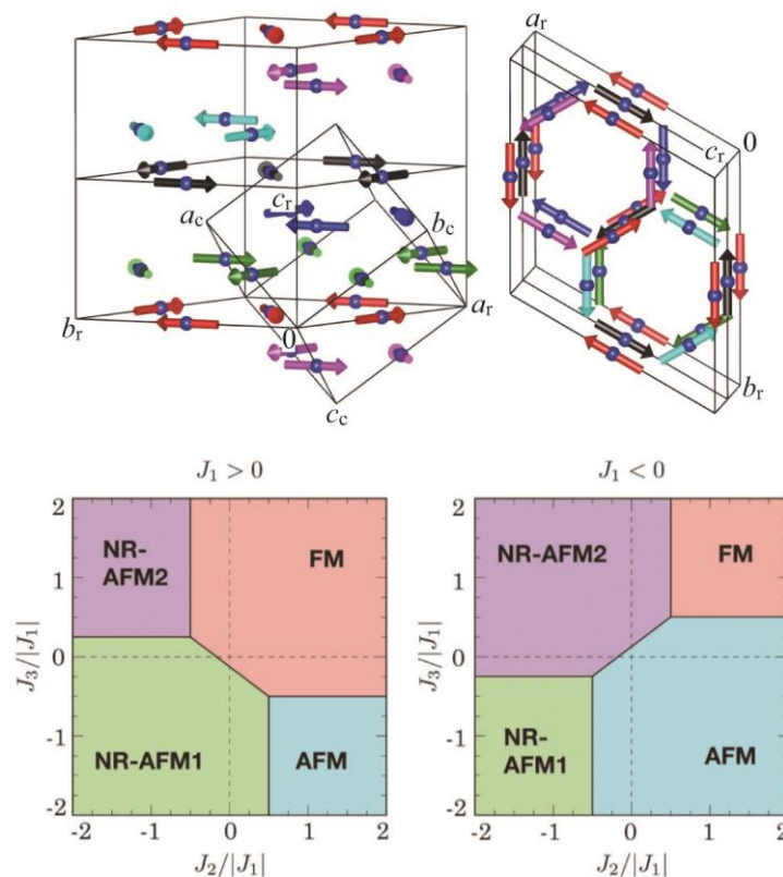
図 1-4 \text{LaMn}_3\text{V}_4\text{O}_{12} の中性子回折により得られた磁気構造(上)と第一原理計算による安定磁気構造解析結果(下)
