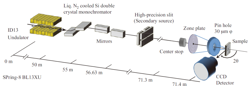
図 3-5 局所構造解析用マイクロX線回折装置
