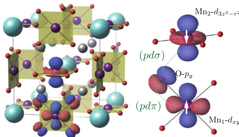
図 4-3 \text{YMn}_3\text{Al}_4\text{O}_{12} の隣接 Mn イオンのスピン間に働く超交換相互作用に寄与する電子軌道の模式図。
