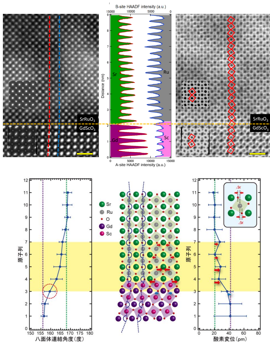
図 1-7 GdScO 3 /SrRuO 3 ヘテロ構造の超高分解能電子顕微鏡環状暗視野(HAADF)・明視野(ABF)像とそのスペクトル解析(上)と酸化物ヘテロ界面近傍における酸素八面体の連結変化
