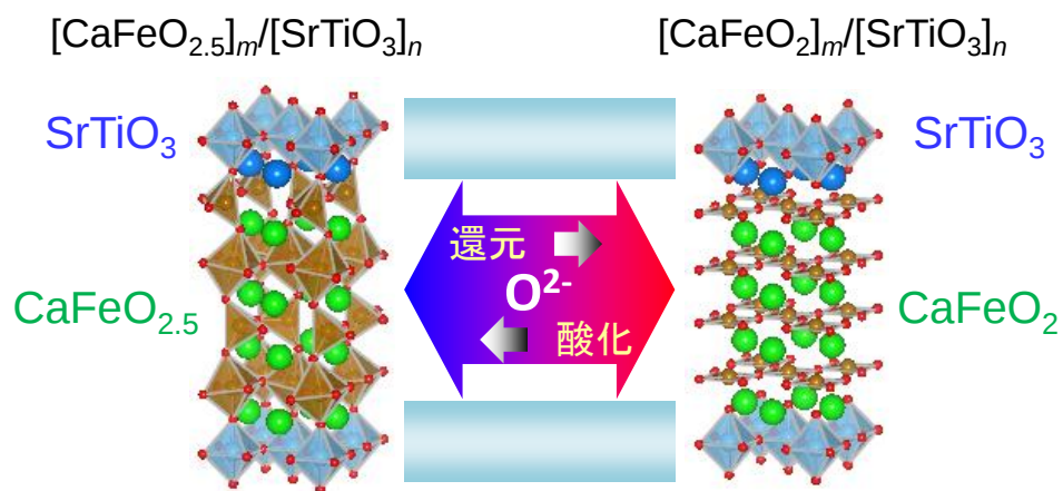
図 1-5 人工超格子薄膜での2次元酸素イオン脱離
