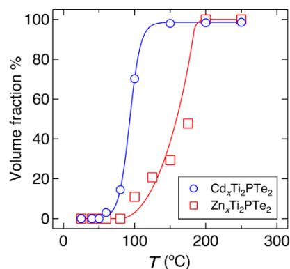
図 2-5 低温における、 Ti_2PTe_2 に対する Cd 、 Zn のインターカレーション反応
