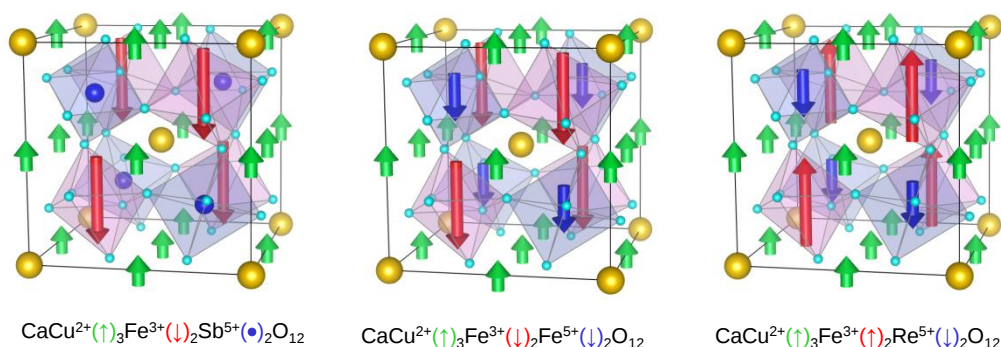
図 3-3 Aサイトペロブスカイト構造酸化物での磁気相互制御
