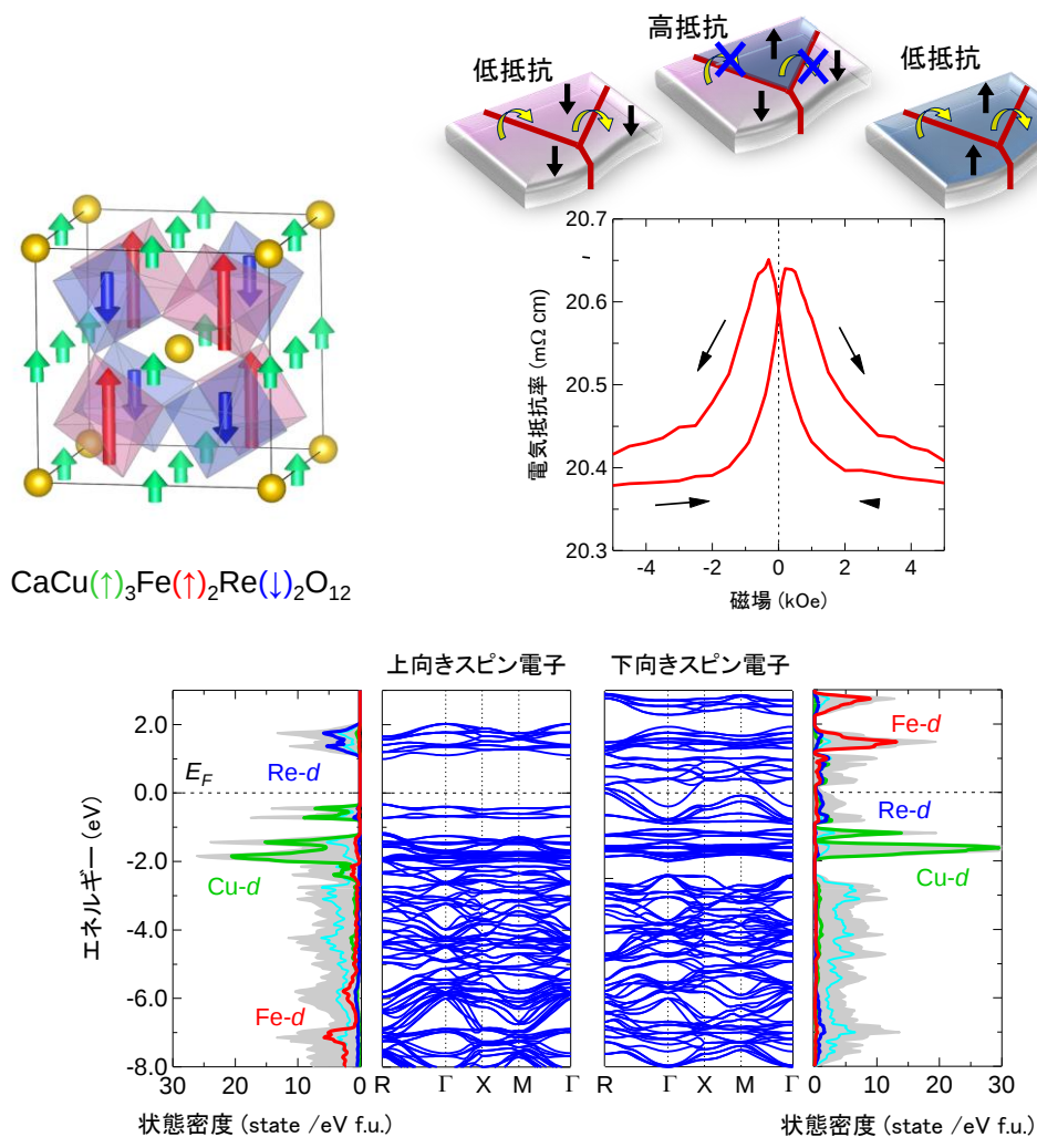
図 1-3 新物質 \text{CaCu}_3\text{Fe}_2\text{Re}_2\text{O}_{12} の結晶・磁気構造(左上)と磁気抵抗効果(右上)、ハーフメタル電子状態(下)
