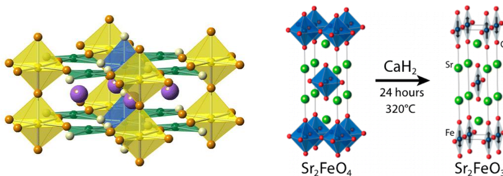
図 2-1 平面4配位ユニットを持つ新物質 \text{BaFeO}_2 (左)と \text{Sr}_2\text{FeO}_3 (の右) 結晶構造
