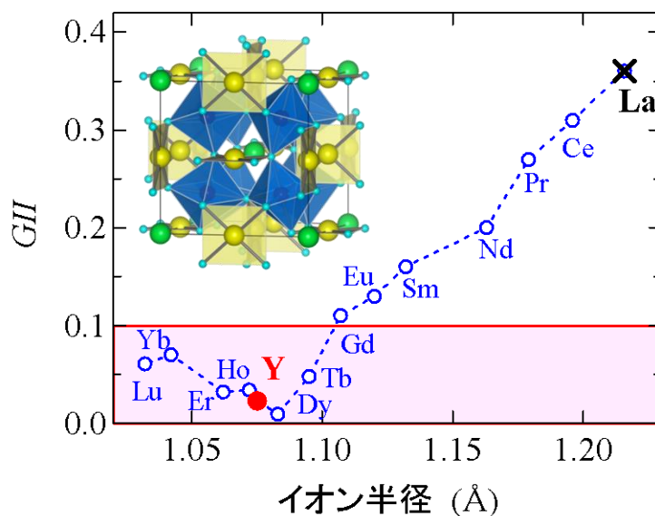
図 1-10 A サイト秩序型ペロブスカイト構造をとる新物質 Ln^{3+}Mn^{2+}_3Al^{3+}_4O_{12} における構造安定性予測
