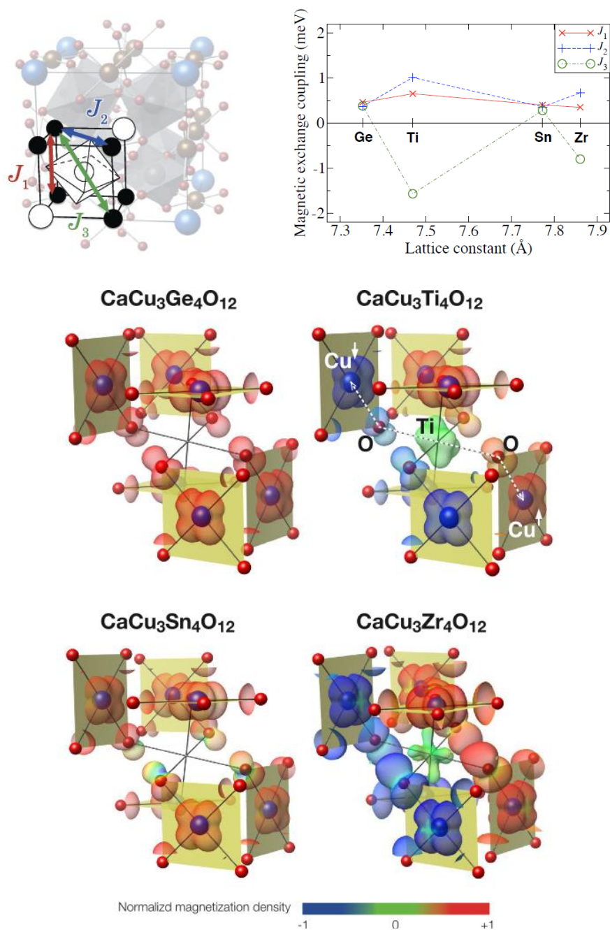
図 4-2 \text{CaCu}_3\text{B}_4\text{O}_{12} でのA' サイトでの磁気相互作用(上)部分電荷密度分布。 \text{CaCu}_3\text{Ti}_4\text{O}_{12} と \text{CaCu}_3\text{Zr}_4\text{O}_{12} では、第三隣接Cuのスピ間に反強磁性的相互作用が働く。
