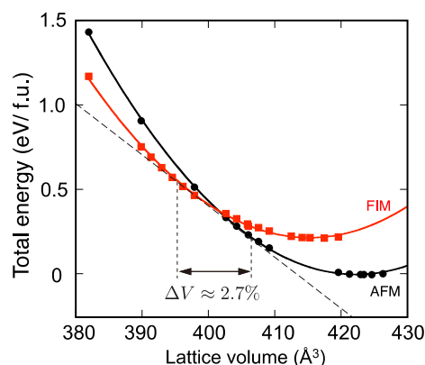
図 4-1 \text{LaCu}_3\text{Fe}_4\text{O}_{12} の絶縁相(黒線、低温で反強磁性秩序を示す)と金属相(赤線、低温でフェリ磁性秩序を示す)の相対安定性の圧力依存性。
