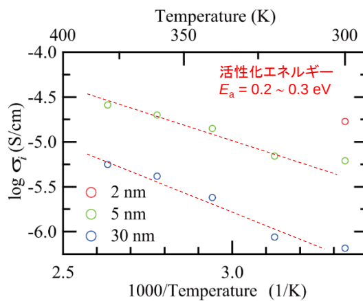
図 1-6 \text{SrFeO}_{2.5} 薄膜の伝導特性
