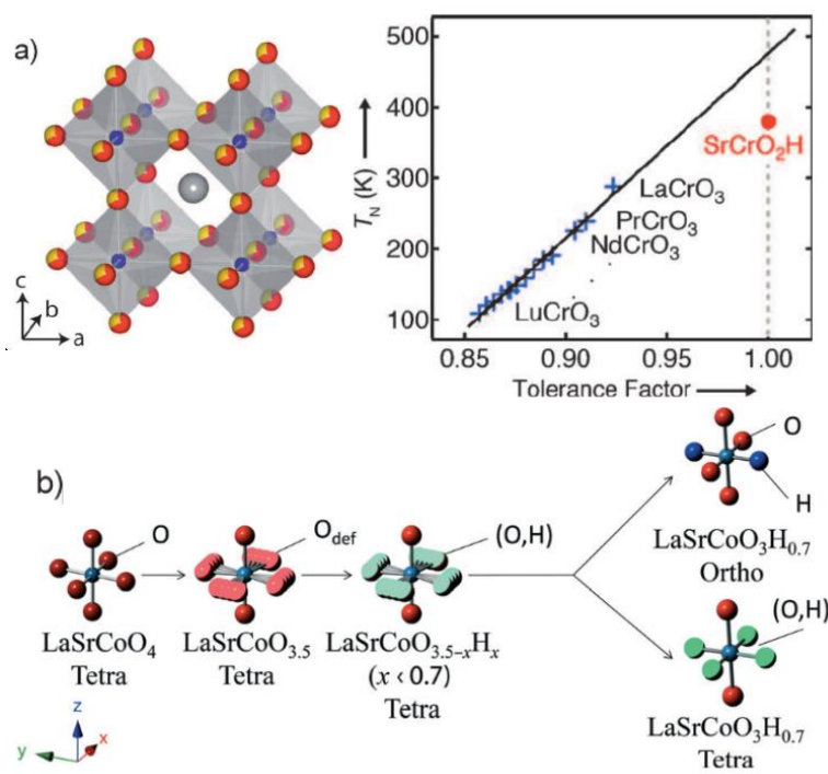
図 2-2 (a) SrCrO 2 H の結晶構造、および磁気転移温度の比較 (b) LaSrCoO 3 H 0.7 における、H - の配位制御
