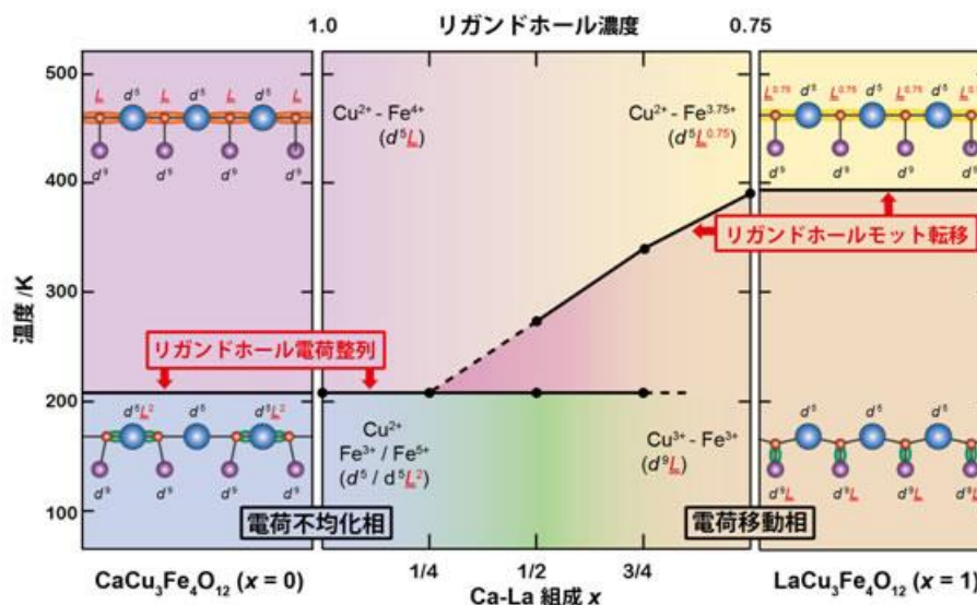
図 1-2 酸素ホールの局在化から見た異常高原子価 Fe イオンの振る舞い
