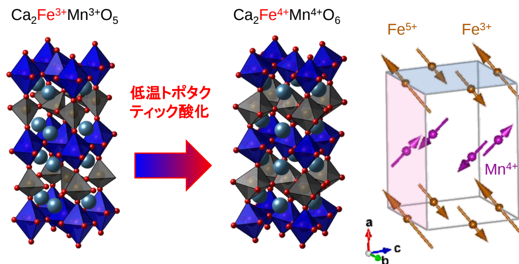
図 1-9 異常高原子価 \text{Fe}^{4+} の 2 次元配列した層状構造 \text{Ca}_2\text{FeMnO}_6 の結晶構造と磁気構造
