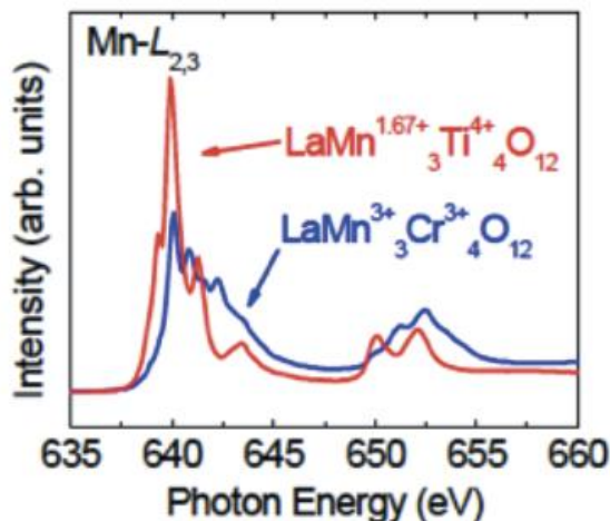
図 3-1 異なる原子価状態における放射光X線 におけるMn-L吸収端スペクトル。
