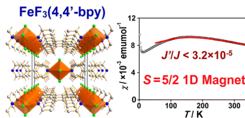
図 2-6 \text{FeF}_3(4,4'\text{-bipy}) の構造と磁性
