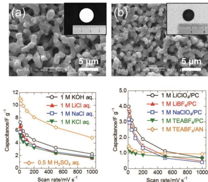
図 2-4 (a) TiO_2 前駆体モノリス、(b) TiN モノリス、(c) 水溶液、および有機溶媒での TiN モノリスのキャパシタ容量
