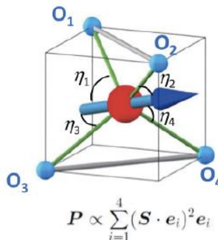
図 4-4 マルチフェロイック物質での電気磁気相互作用
