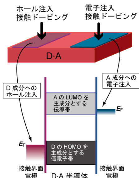
図 25 中性電荷移動錯体 D-A への接触ドーピングによって作製される素子
