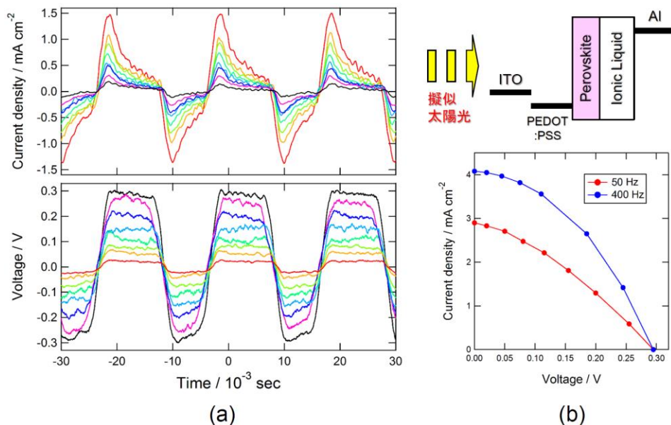
図20 [ITO|Perovskite|IL|Al] なる構造をもつ光電セルの光-交流電気エネルギー変換。(a) 50 Hz チョップ光から生じる交流電流 (上) と電圧 (下)。(b) 電流-電圧曲線 (50 および 400 Hz)。
