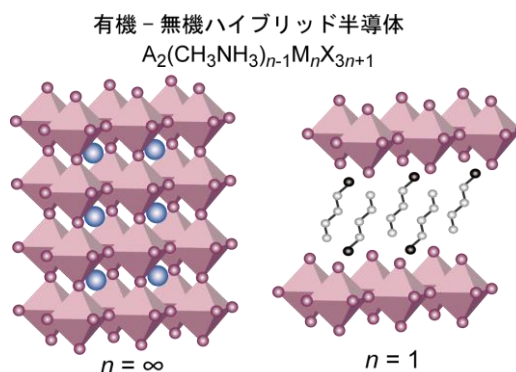
図 21 有機-無機ハイブリッド金属ハロゲン化物の構造
