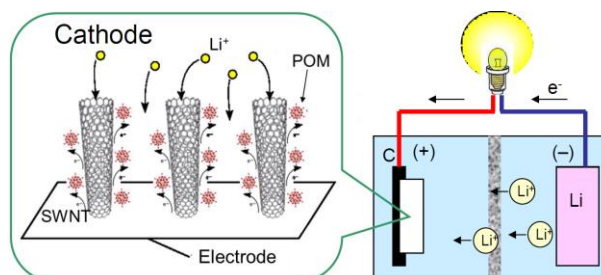
図 2 分子クラスター電池の概念図
