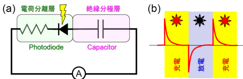
図 11 (a) BDTDA 光電セルの簡易化した等価回路。電極界面の「電荷分離層」と薄膜内部の「絶縁分極層」を、それぞれフォトダイオードとコンデンサで表している。(b) 等価回路を見ても分かるように、コンデンサでは、光照射時に充電、光遮断時に放電が生じる。
