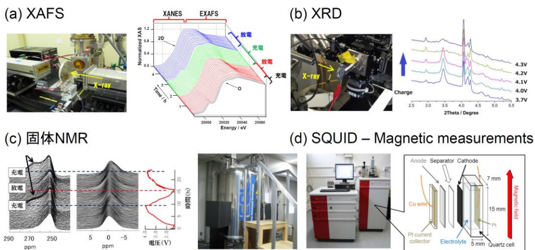
図 3 本研究により立ち上げたさまざまな電気化学 operando 計測システム。
