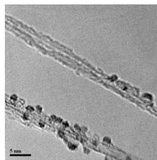
図 4 POM-SWNT ナノハイブリッドの TEM 像。黒いドットが個別分離吸着した POM 分子。
