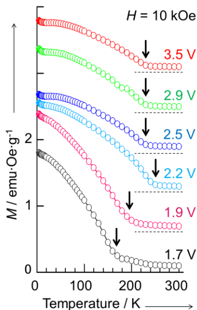
図8 固体電気化学反応中の Cr(II)- Cr(III) PBA の磁化の温度依存性。矢印は転移温度 T_{No} 。
