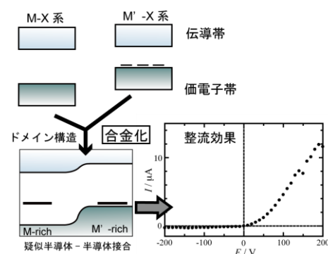
図 23 有機・無機ハイブリッド金属ハロゲン化物の合金化によって形成される疑似半導体接合
