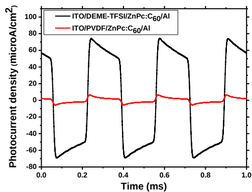
図 14 [\text{ITO} | \text{ZnPc}\cdot\text{C}_{60} | \text{PVDF} | \text{Al}] と [\text{ITO} | \text{ZnPc}\cdot\text{C}_{60} | \text{DEME-TFSI} | \text{Al}] 光電セルからの光電流。
