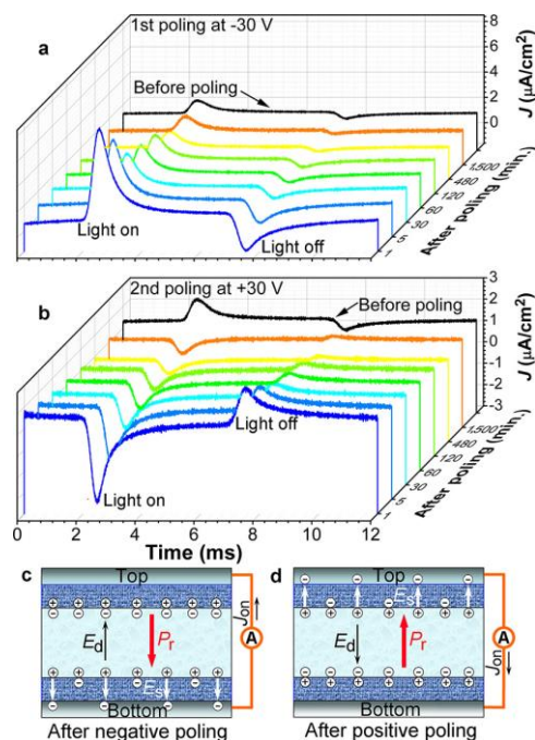
図 19 分極した[Al | CuPc | P(VDF-TrFE) | CuPc | Al]セルから得られた過渡光電流の時間変化。
