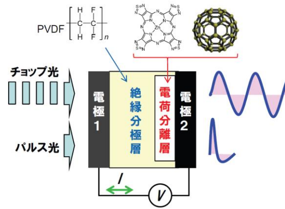
図 12 本研究で提案する[電極1 (M) | 絶縁分極層 (I) | 電荷分離層 (S) | 電極2 (M)] (= MISM) 構造。チョップ光を交流に高効率変換し、パルス光を超高速変換する。
