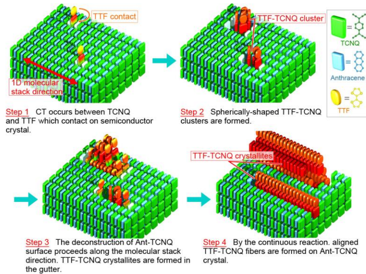
図 27 交互積層型中性 TCNQ 電荷移動錯体結晶表面上への TTF 蒸気接触による一次元配向 TTF-TCNQ 薄膜形成過程の模式図
