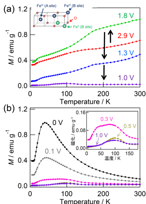
図9 固体電気化学反応中の \text{Fe}_3\text{O}_4 の磁化の温度依存性。(a) 2.9 \sim 1.0 V における変化。挿入図は \text{Fe}_3\text{O}_4 の構造。(b) 1.0 \sim 0 V における変化。挿入図は拡大図。
