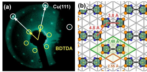
図 29 (a) BDTDA/Cu(111) の LEED パターン. (b) Cu(111) 基板上で予想される BDTDA の配列。グレーの三角グリッドは Cu(111)格子、オレンジと緑のひし形はそれぞれ Cu(111) と BDTDA の単位格子を表す。オレンジのドットはイオウ原子を示している。
