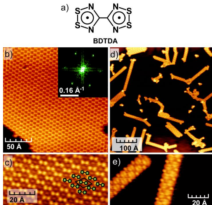
図 28 (a) BDTDA の分子構造。(b) Cu(111)基板上に BDTDA がつくる 2 次元ハニカム構造 ( 200 \times 200 \text{ Å}^2 , 100 pA, -0.8 V, 80 K)。挿入図はフーリエ変換イメージ。(c) (b)と同様(ただし、 80 \times 40 \text{ Å}^2 , 50 pA, -0.8 V, 80 K)。(d) Ag(111) 基板上に BDTDA がつくる 1 次元ナノリボン構造 ( 500 \times 500 \text{ Å}^2 , 100 pA, -2 V, 80 K)。(e) (d)と同様(ただし、 100 \times 50 \text{ Å}^2 , 140 pA, -0.1 V, 80 K)。
