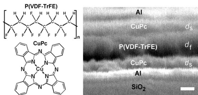
図 18 有機強誘電体をサンドイッチした光電セルの構造。スケールバーの長さは 100 nm。
