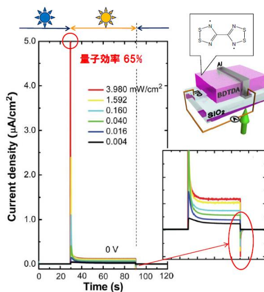
図 10 [ITO | BDTDA(300 nm) | Al] 光電セルへの光照射 (532 nm) によって得られた巨大過渡電流。挿入図は拡大図で、光遮断直後には負のスパイク電流も観測される。
