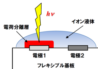
図 17 新しい有機光電セルの構造。
