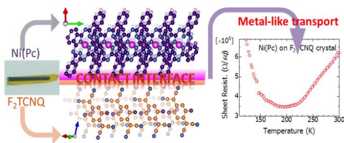
図 26 \text{Ni(Pc)} 単結晶と \text{F}_2\text{TCNQ} 単結晶の貼り合わせによる界面の高伝導化
