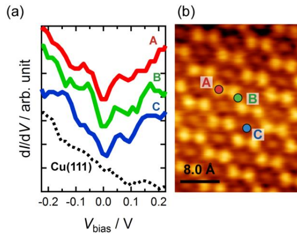
図 30 BDTDA/Cu(111)のSTS像。(a) -0.2 \sim 0.2 Vにおける dI/dV 曲線。A, B, C はパネル(b)での測定箇所を示している。点線はクリーン Cu(111) 面の STS 像。
