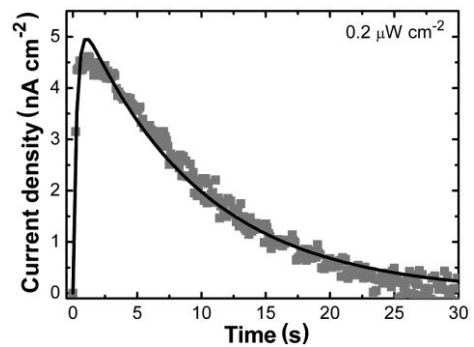
図 13 [ITO|BDTDA|Al]セルに生じる過渡光電流の起源とその時間依存。実線は理論曲線。
