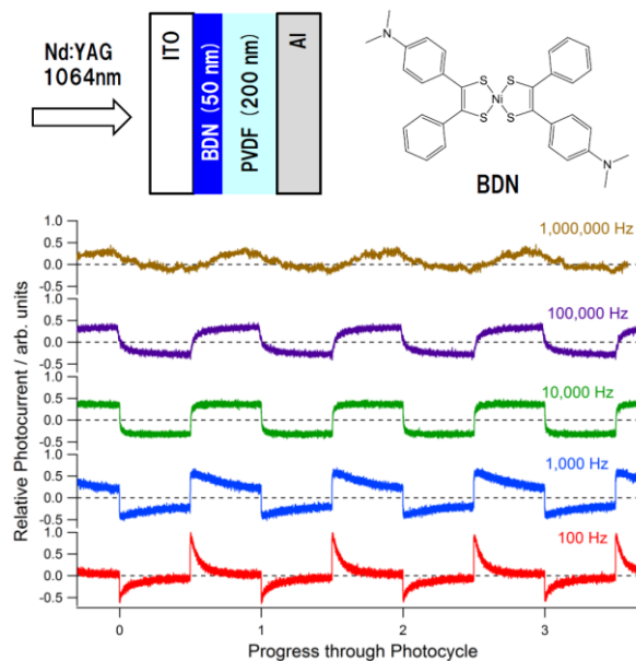
図 15 BDN 光電セルの構造と、Nd:YAG 近赤外光パルス(1064 nm, 1 ns)に対する光電流変換。
