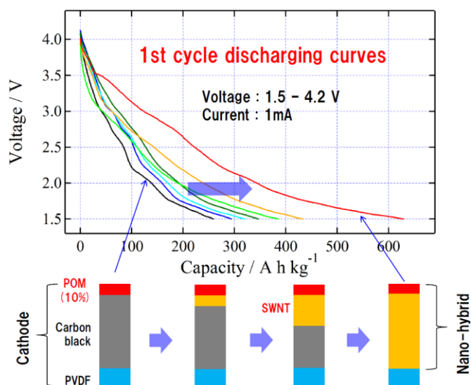
図 5 POM-SWNT ナノ複合体を活性物質とする分子クラスター電池の第一放電曲線。
