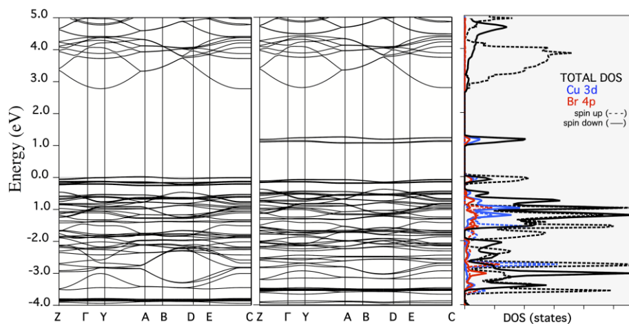
図 24 (\text{PTA})_2\text{CuBr}_4 のバンド構造と状態密度。バンド構造図左は up-spin、右は down-spin を示す
