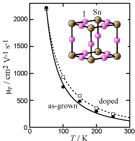
図 22 Hall 効果測定によって得られた \text{CH}_3\text{NH}_3\text{SnI}_3 単結晶試料の移動度の温度変化
