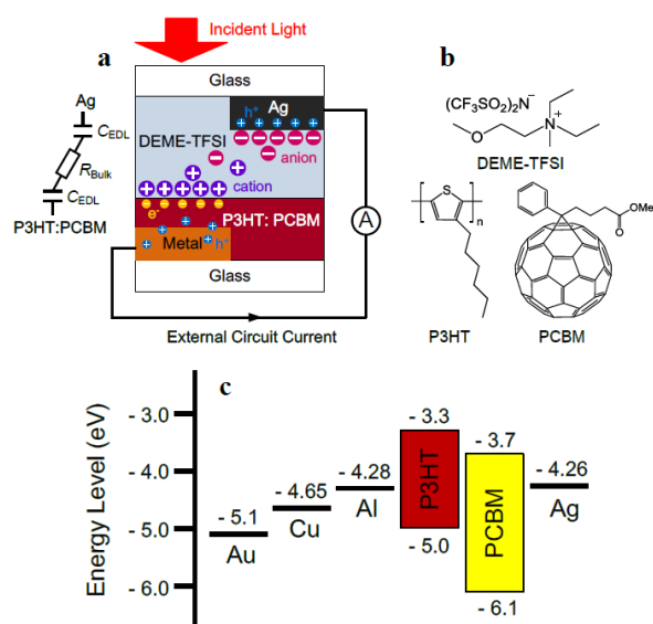
図 16 (a) 透明電極を全く用いない光電セルの設計。(b) 構成成分の分子の構造。(c) 分子の軌道エネルギーと電極の仕事関数。
