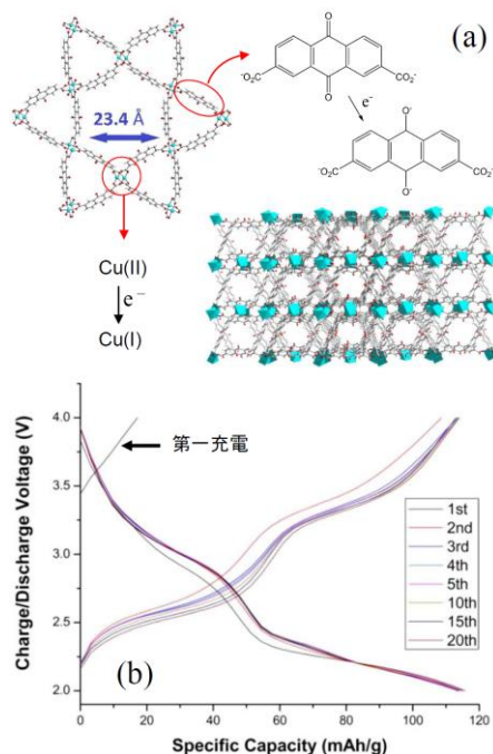
図7 レドックス活性 MOF [Cu(2,7-AQDC)(DMF)] n の結晶構造 (a) と、これを正極活物質とする Li 電池の充放電曲線 (b)。
