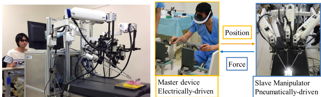
図 3.2.6 試作した力覚提示機能を有するマスタ・スレーブ型手術支援ロボットシステム
