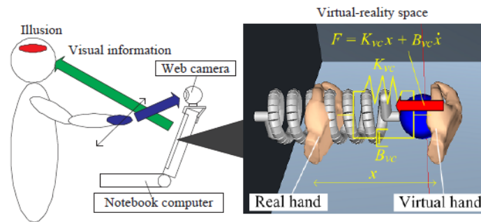
図 3.2.1 バーチャルカップリングを用いた疑似力覚提示装置の概要
