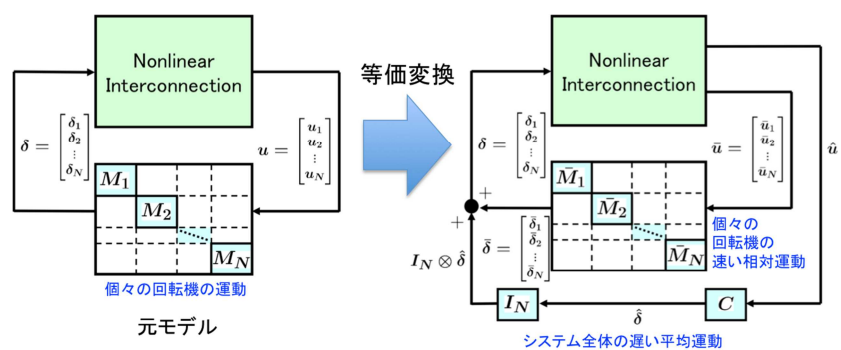
図 3-3: 電力システムに生起するダイナミクスの階層的表現. 左の N 機の回転機に対する元モデルより等価な右のモデルを導出する. N 機の回転機の速い相対運動とシステム全体の遅い平均運動との関係を陽に表現している. 本研究では上記の階層的表現に基づいてシステムの安定条件を導出した。
