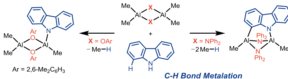
スキーム 3-2-5. アルミニウム二核錯体による炭素—水素結合のメタル化反応
