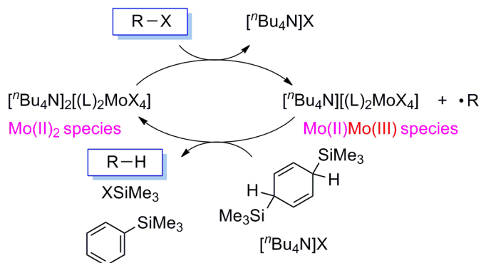
脱ハロゲン化の反応機構
